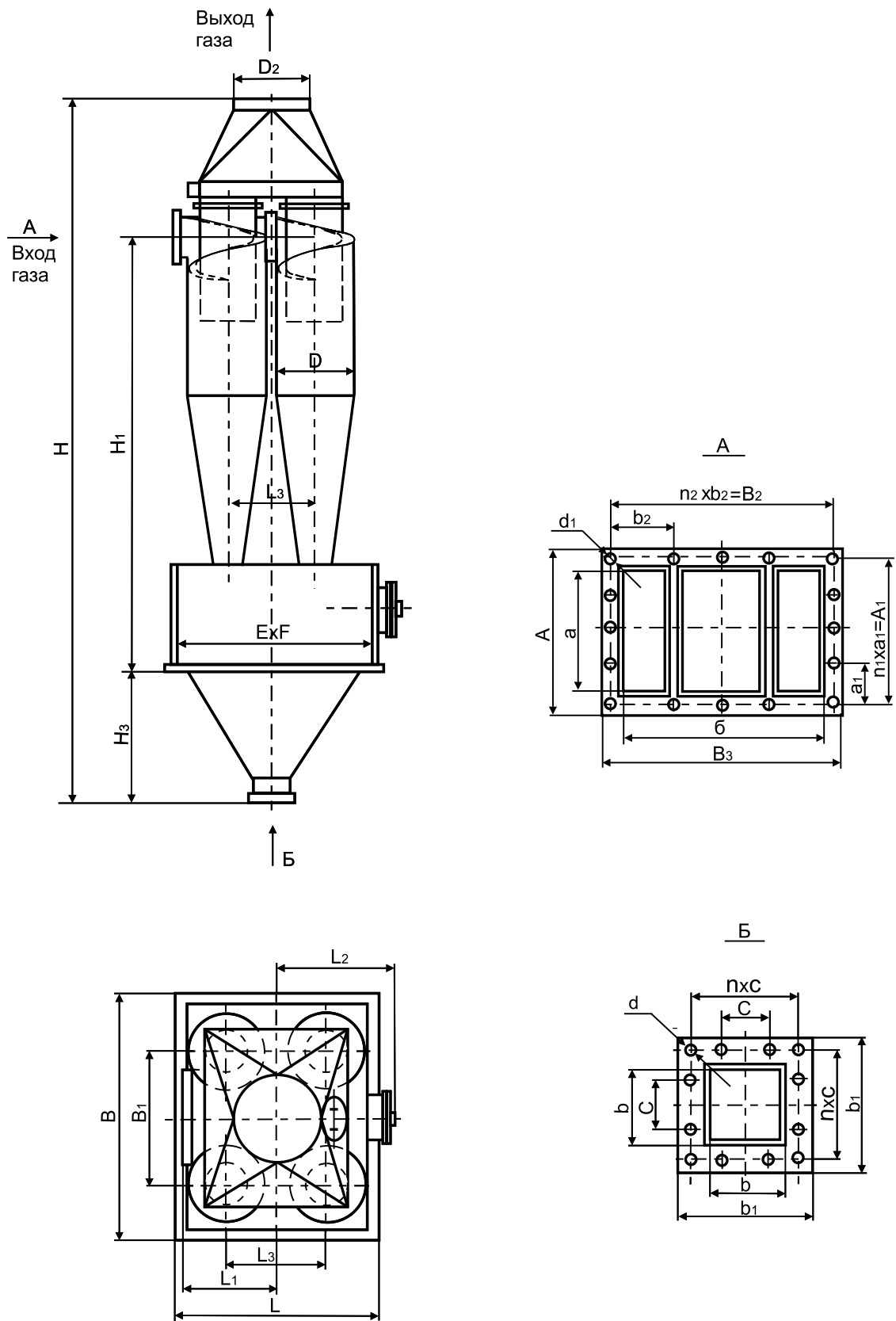
Рис.7 Циклон типа ЦН-15x4СП
