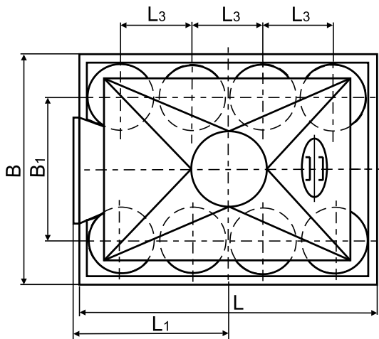
Рис.9 Циклон типа ЦН-15х4СП
