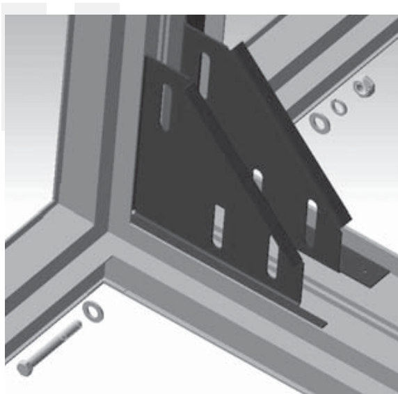
Рис. 6 Крепление секций при помощи внутренних уголков
