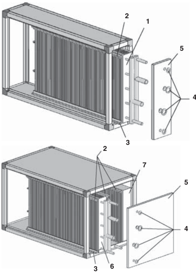
Рис. 11 Разборка секций с теплообменниками
