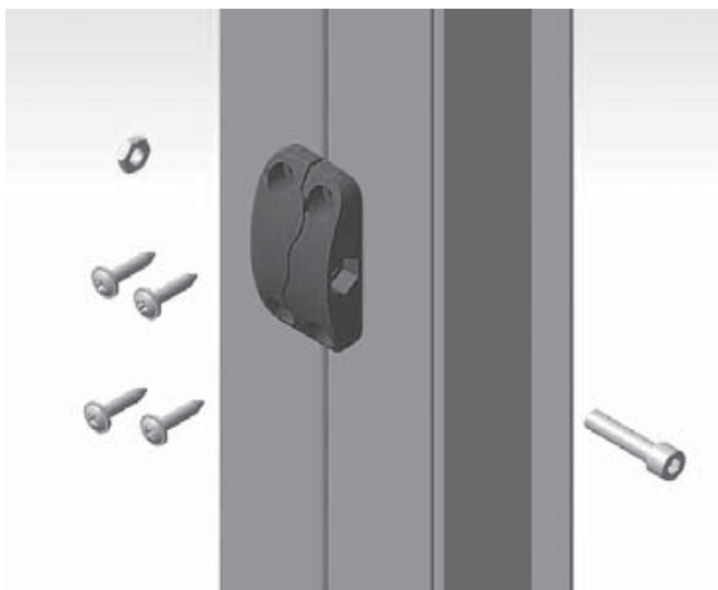
Рис. 5 Крепление наружной межсекционной стяжки
