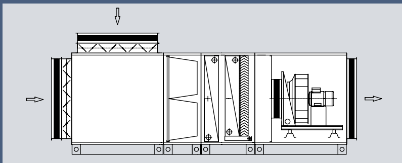
6) Установка для подачи воздуха со смешиванием, фильтрацией, водяным нагревом, охлаждением
