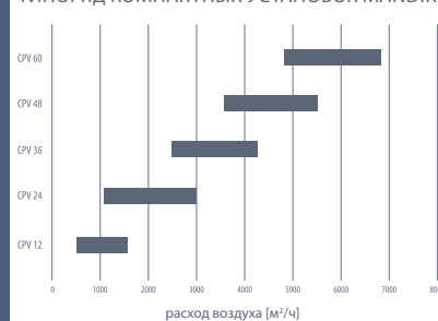
ТИПОРАД КОМПАКТНЫХ УСТАНОВОК MANDÍK
