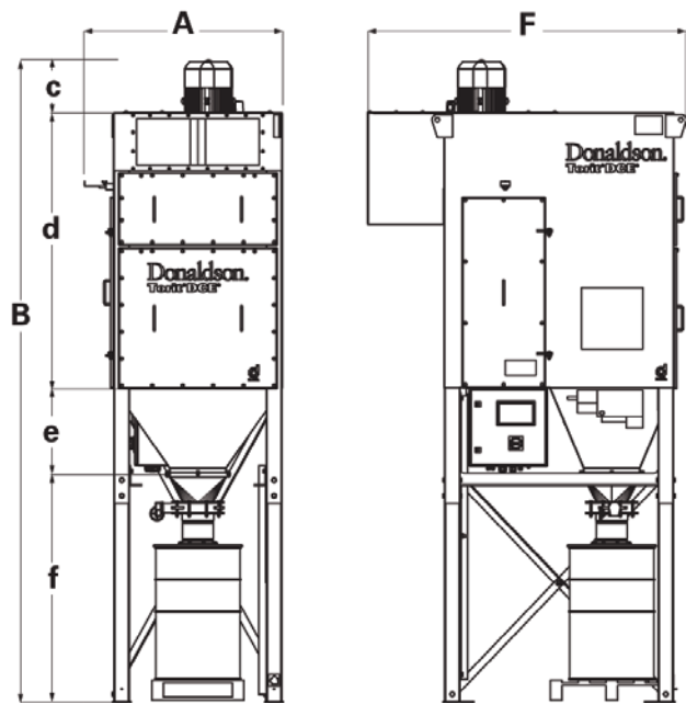
ЧАСТИЧНО ВСТРОЕННЫЙ ВЕНТИЛЯТОР
