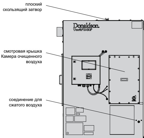
БОКОВАЯ ПРОЕКЦИЯ
