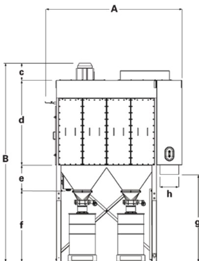
ЧАСТИЧНО ВСТРОЕННЫЙ ВЕНТИЛЯТОР
