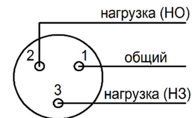
Вариант подключения с разъемом ШР20ПЗЭШ7
