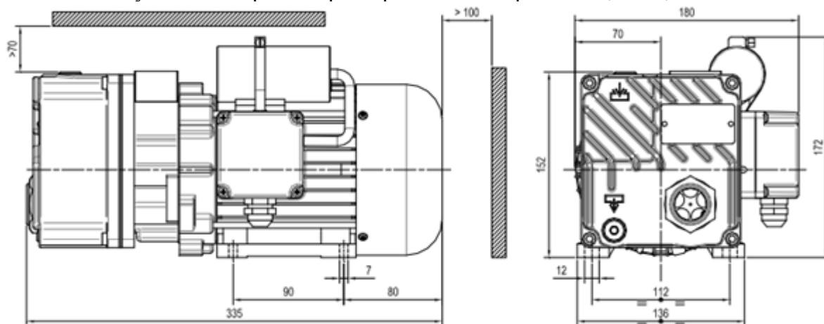
Рисунок 1. Габаритные размеры насосов серий: LB.2, LB.3, LB.4
