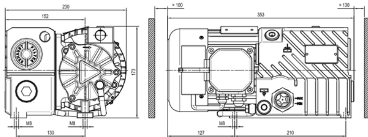
Рисунок 4. Габаритные размеры насосов серии: LB.18
