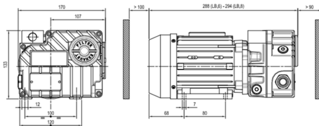
Рисунок 2. Габаритные размеры насосов серии: LB.5
