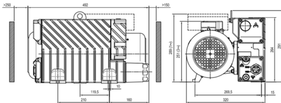
Рисунок 4. Габаритные размеры насосов серии: LB.18
