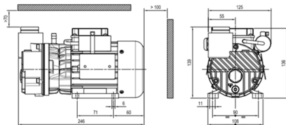
Рисунок 1. Габаритные размеры насосов серий: LB.2, LB.3, LB.4
