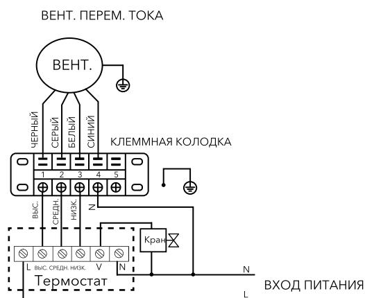
Принципиальная электрическая схема (ВЕНТ. ПЕРЕМ. ТОКА)
