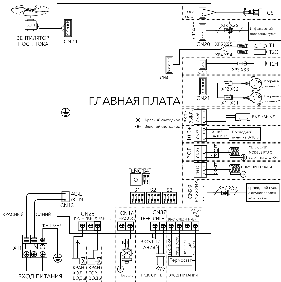
Принципиальная электрическая схема (ВЕНТ. ПОСТ. ТОКА)
