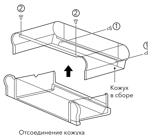
Отсоединение кожуха
