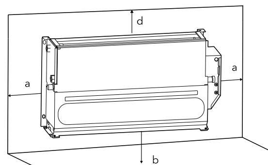
Вертикальная установка снаружи
