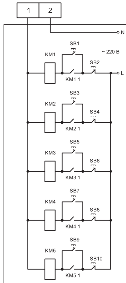
Схема А5 для ЭНП-5
