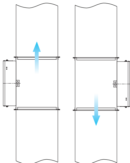
Рисунок 5.3 – Варианты монтажа
