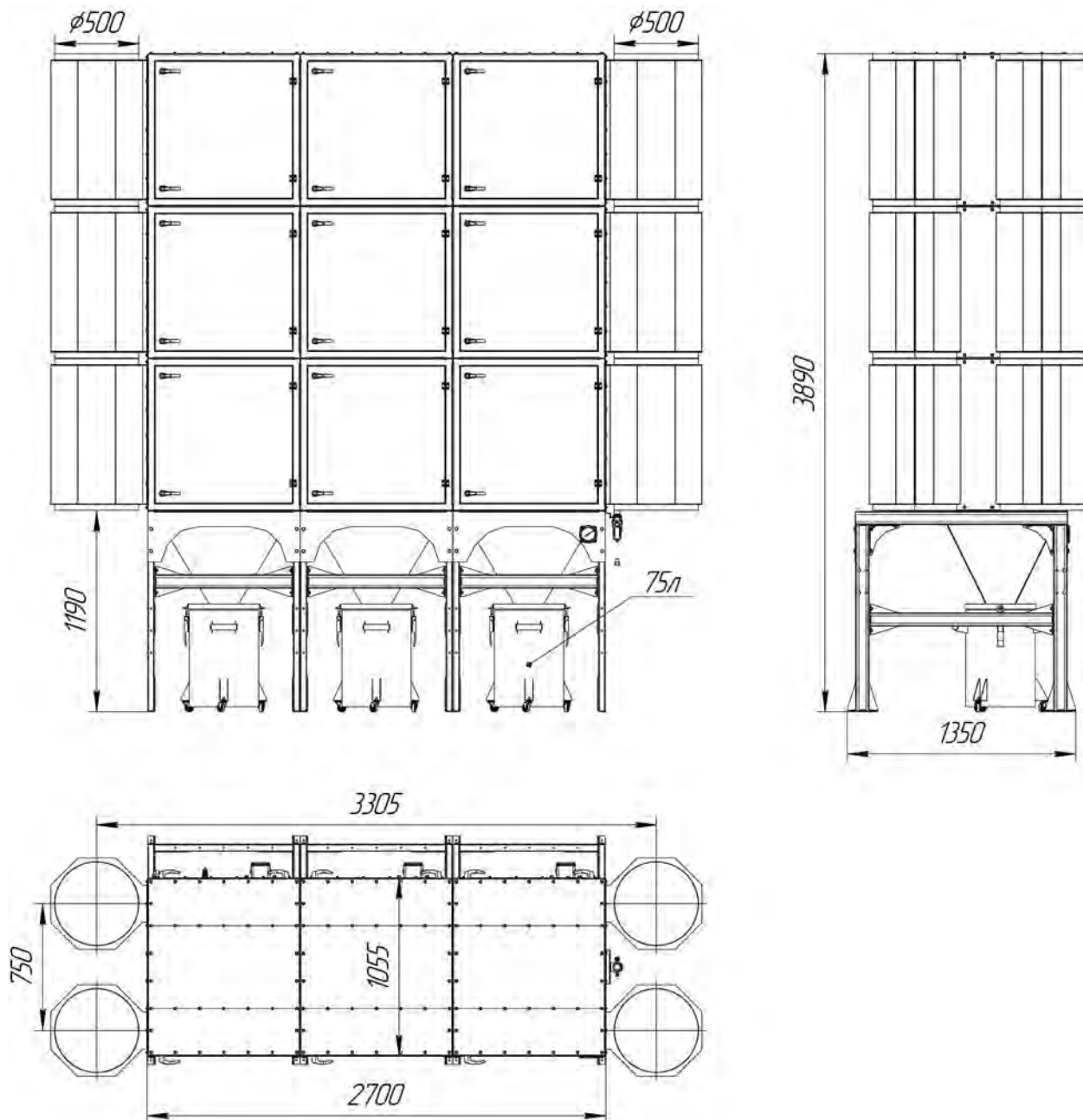
Рис. 37 FCS-ECO-36
