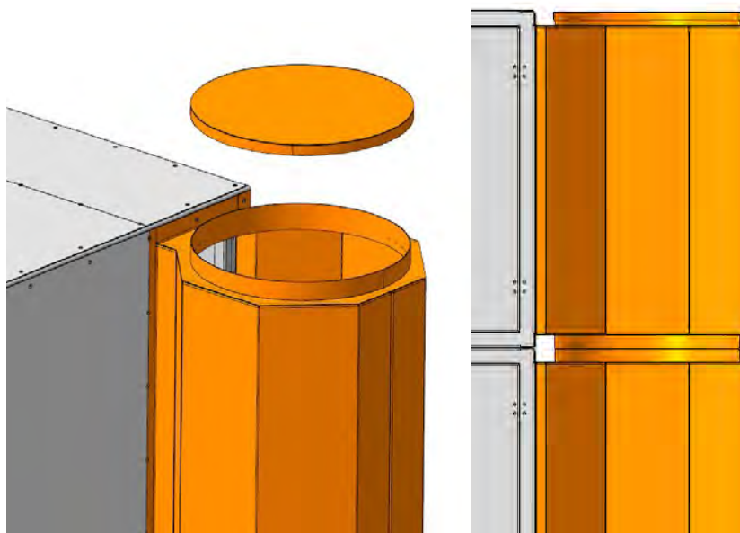
Рис. 10. Установка заглушки
