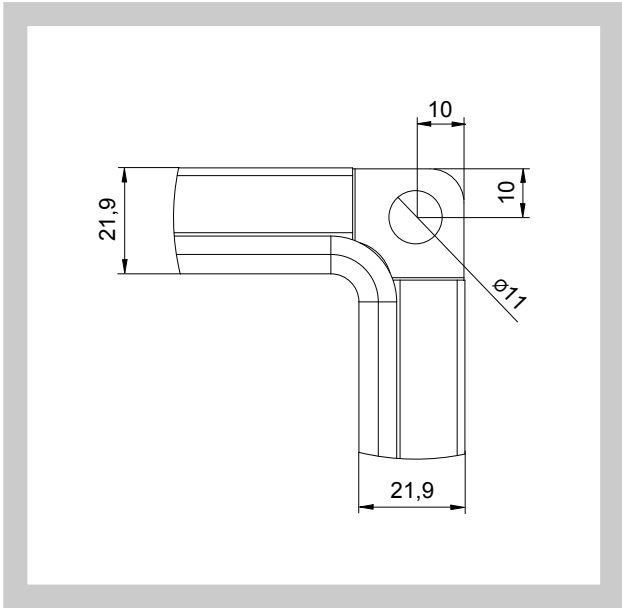
Fig. 5 Corner flange 20 mm
