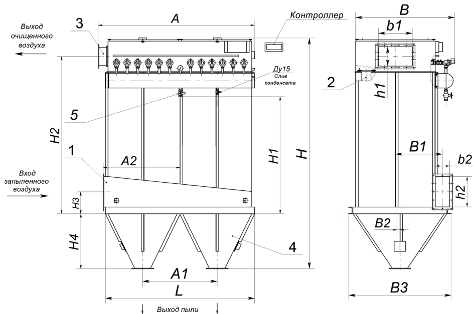
Рис.3 Схема фильтров рукавных типа ФРИП-60; ФРИП-270; ФРИП-360 1 - выходной патрубок; 2 - фильтрующий рукав; 3 - входной патрубок; 4 - бункер; 5 - патрубок для подключения сжатого воздуха.
