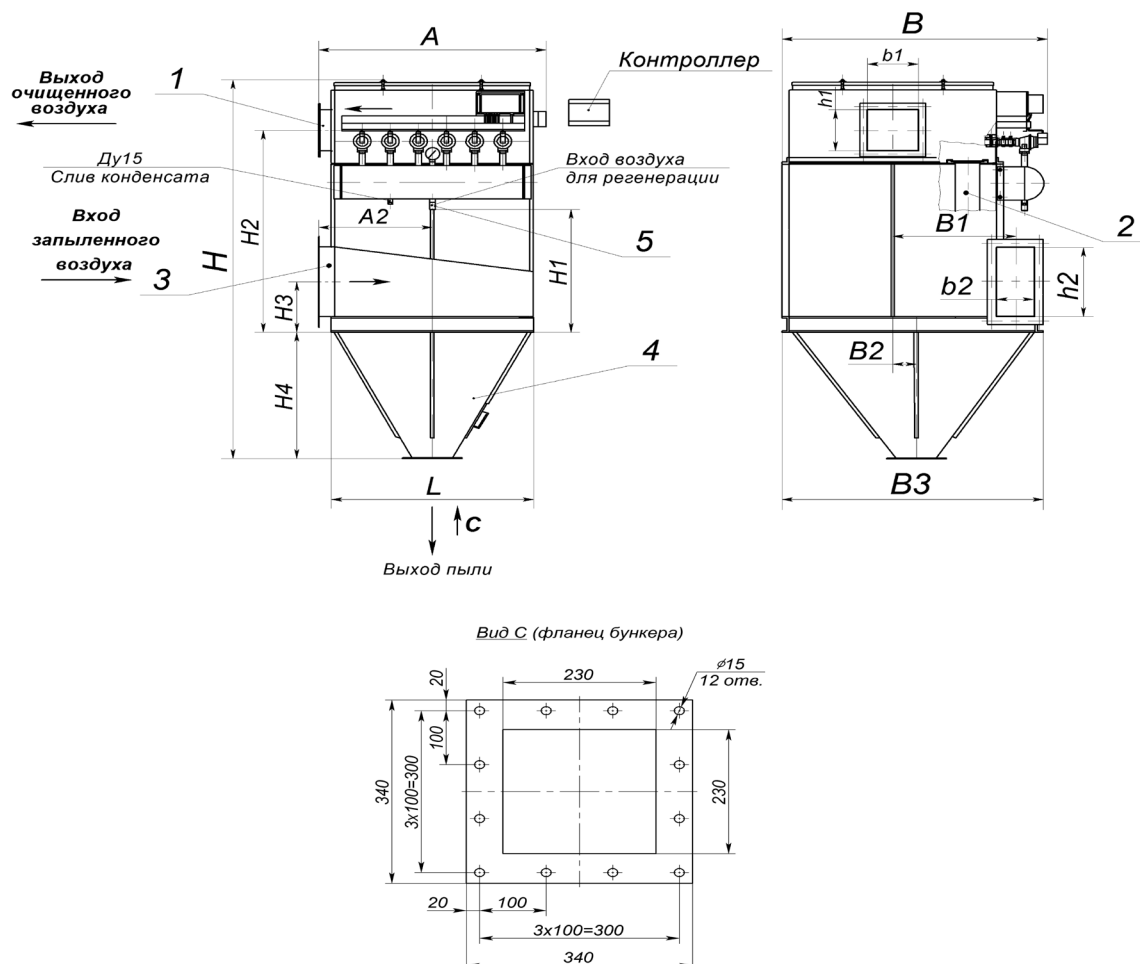
Рис.2 Схема фильтров рукавных типа ФРИП-5; ФРИП-10; ФРИП-15; ФРИП-30; ФРИП-180 1 - входной патрубок; 2 - фильтрующий рукав; 3 - выходной патрубок; 4 - бункер; 5 - патрубок для подключения сжатого воздуха.
