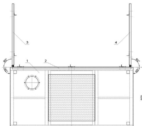
Рис. 4 Схема раскрытия защитных панелей стола сварщика 1 – корпус стола сварщика; 2 - неподвижная защитная панель; 3 – подвижная защитная панель (левая); 4 – подвижная защитная панель (правая).
