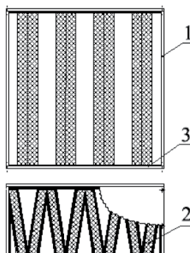
Рис.2 Схема фильтра ФяС-F-МП
