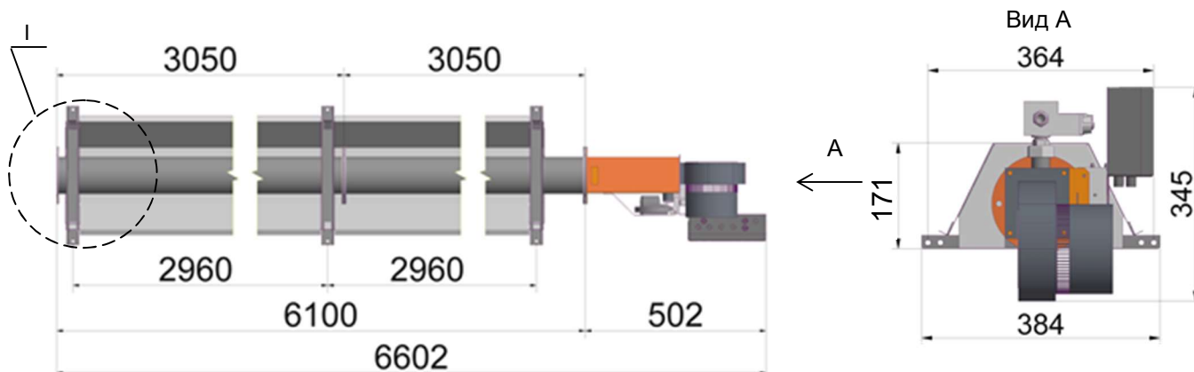
ГИИ-ТМ-15/20 L
