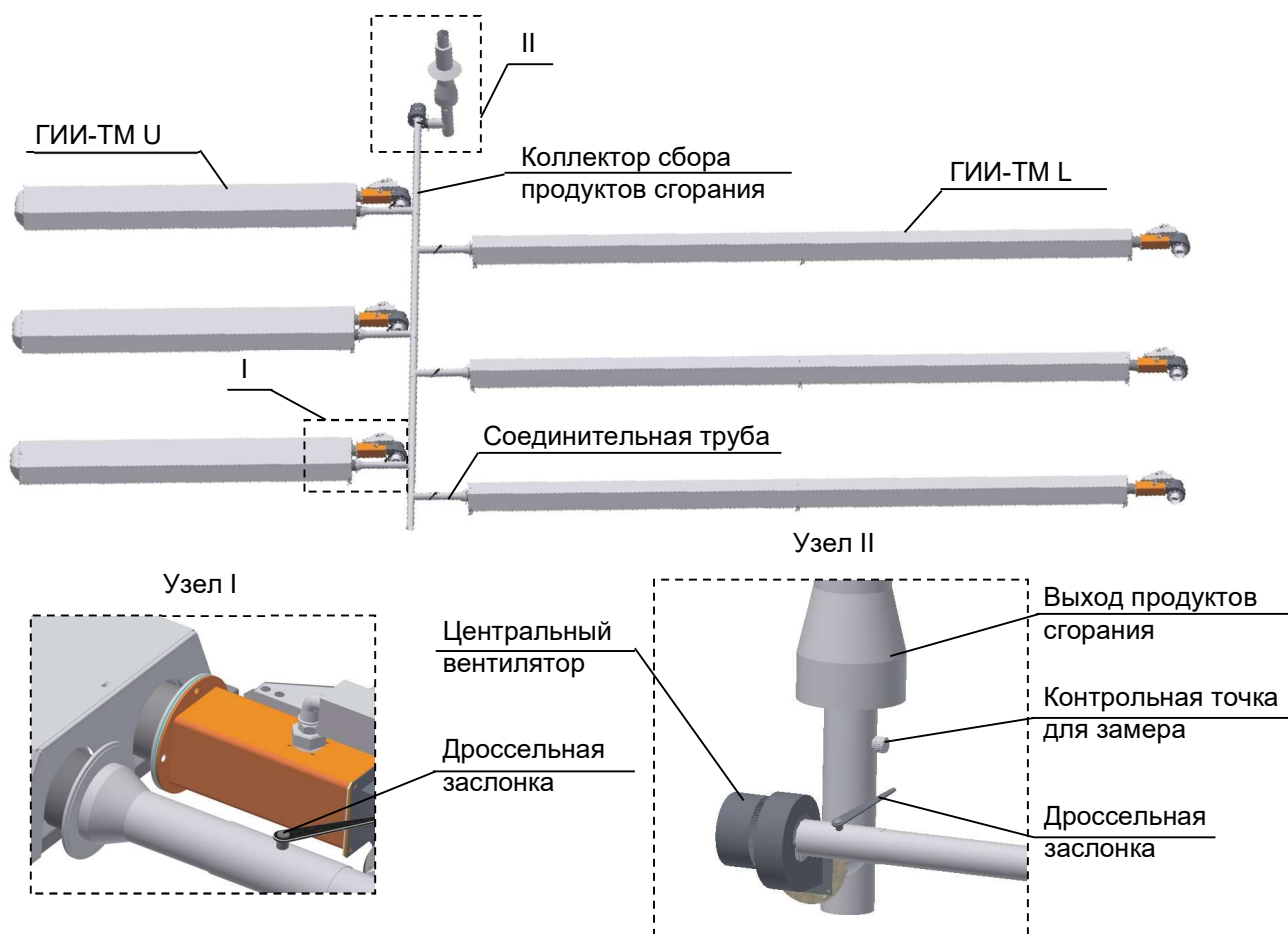
Рисунок 6.2.2 Коллекторная система отвода продуктов сгорания
