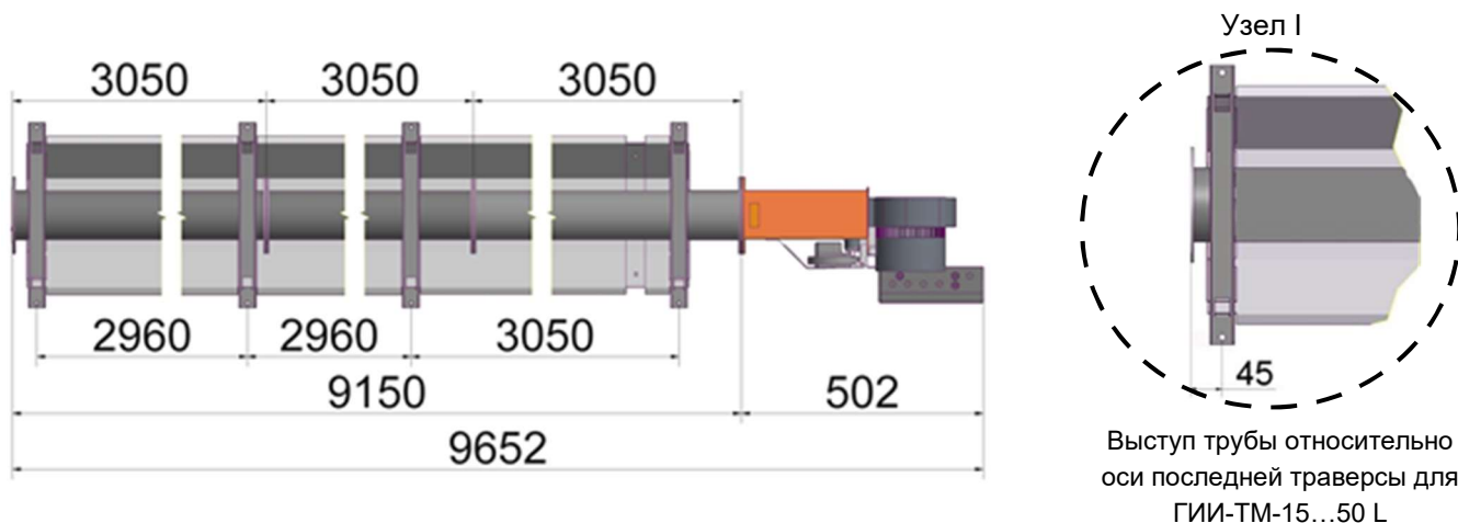
ГИИ-ТМ-40 L
