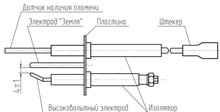
Рисунок 4.5.1 Свеча зажигания
