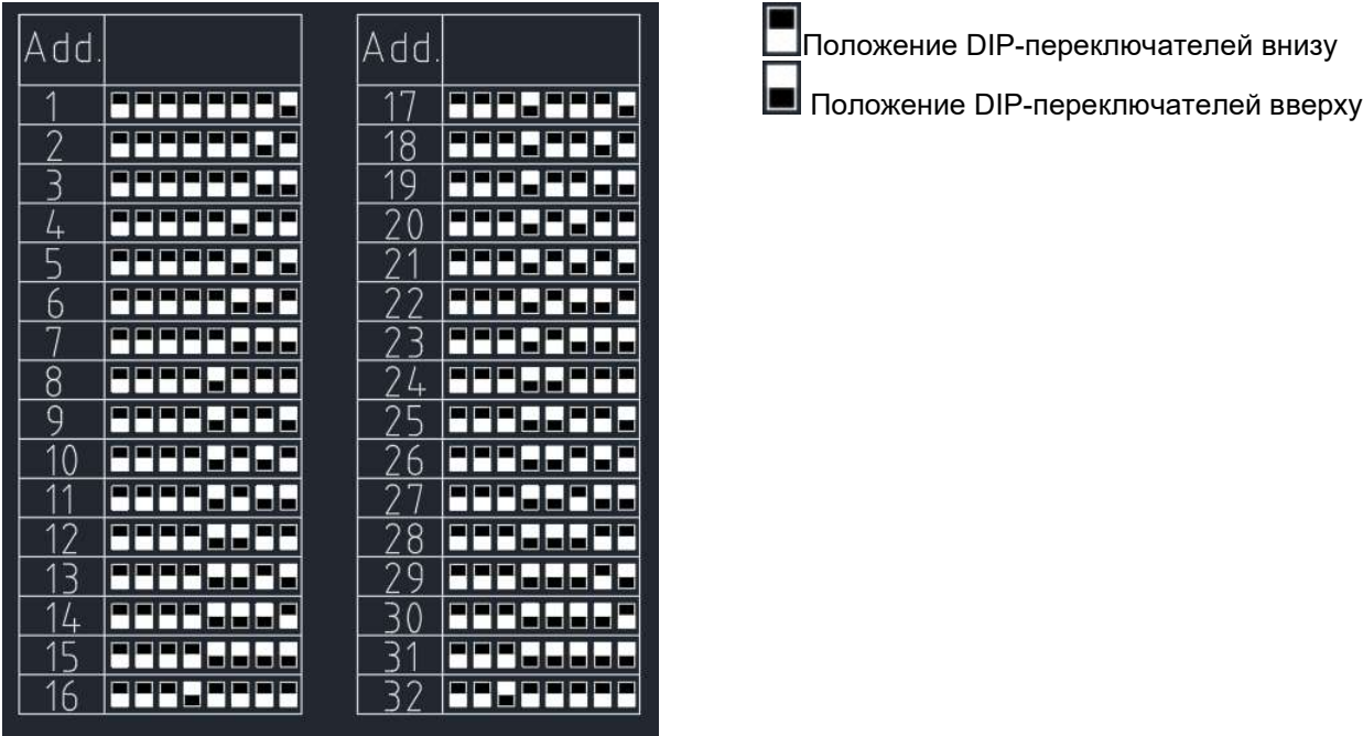
Рисунок 5.3.1 Адресация Modbus IC 4000/1 через DIP переключатели
