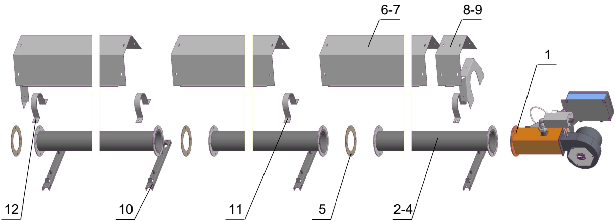
Рисунок 14.1 Запасные части излучателя ГИИ-ТМ L
