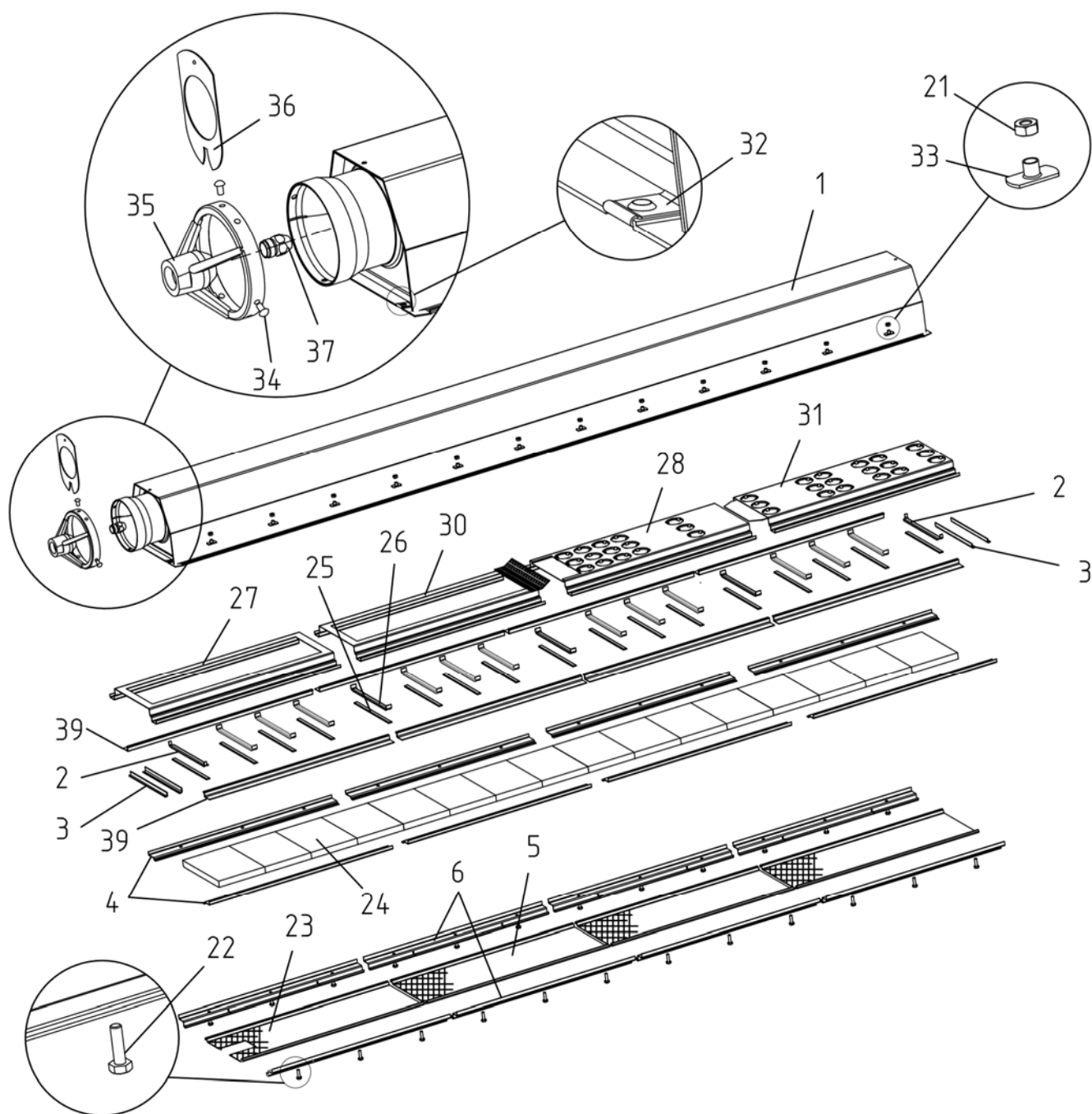
Рисунок 13.1 Запасные части для ГИИ-30/40. Блок горелки
