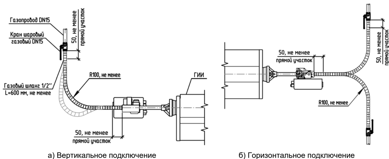
Рисунок 6.2 Подключение излучателя к газопроводу
