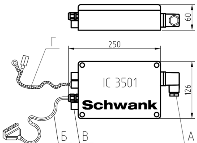
Рисунок 4.3.1 Устройство розжига и контроля горения IC 3501. Внешний вид
