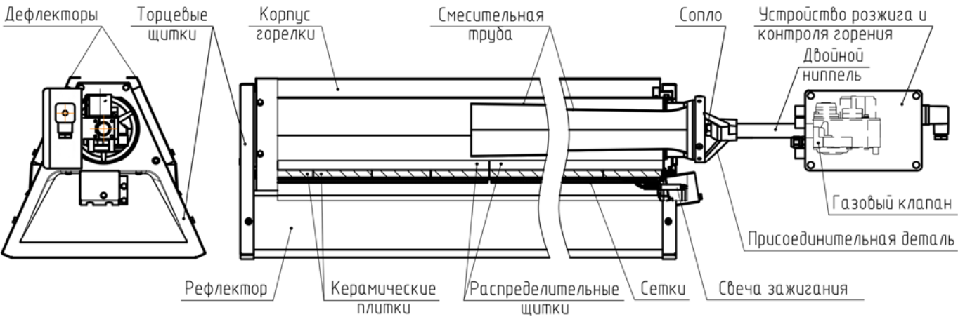
Рисунок 4.1.1 Устройство излучателя
