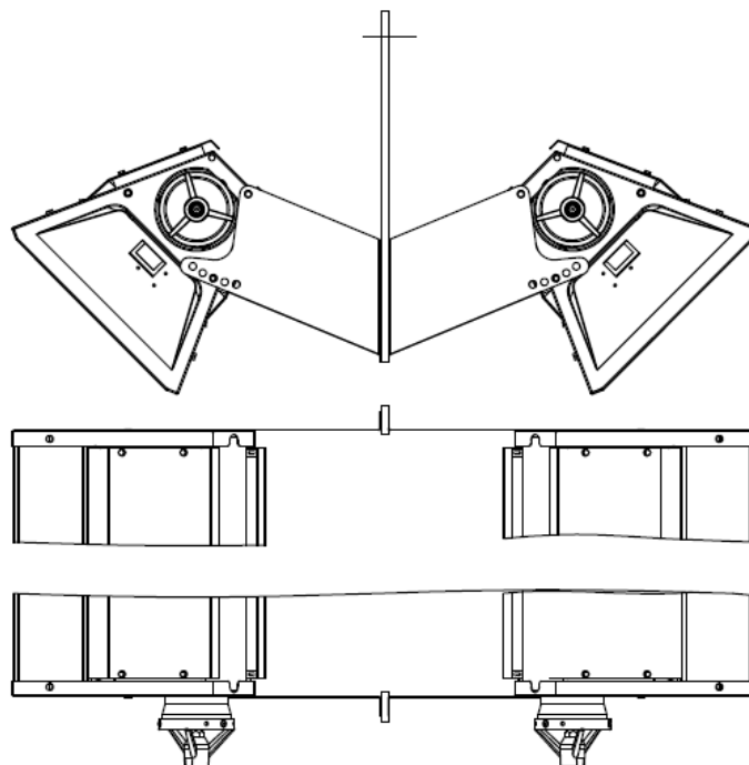
Рисунок 6.6 Двухстороннее крепление на консолях
