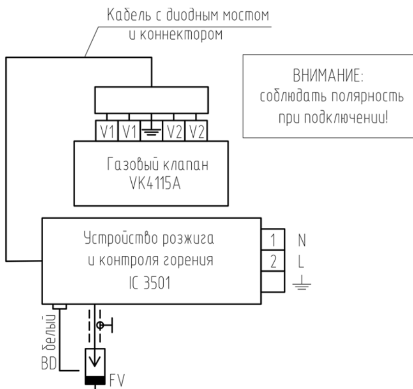
Рисунок 5.2 Электрическая схема подключения
