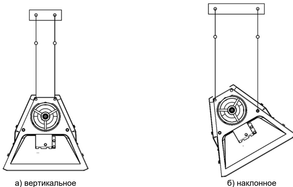
Рисунок 6.7 Крепление на цепях/тросах
