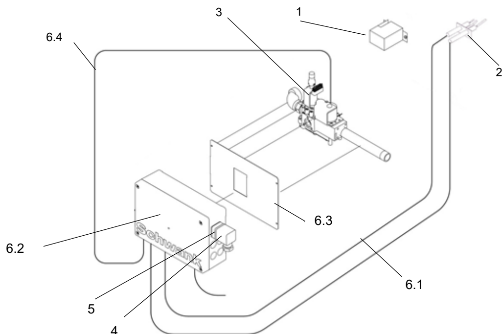
Рисунок 13.2 Запасные части автоматики ГИИ с IC 3501
