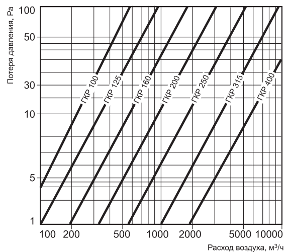
ГРАФИК АЭРОДИНАМИЧЕСКИХ ХАРАКТЕРИСТИК ГКР длиной 900 мм
