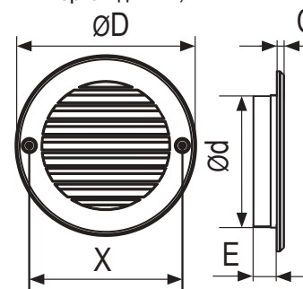
Чертеж для РК, ARK и РКН
