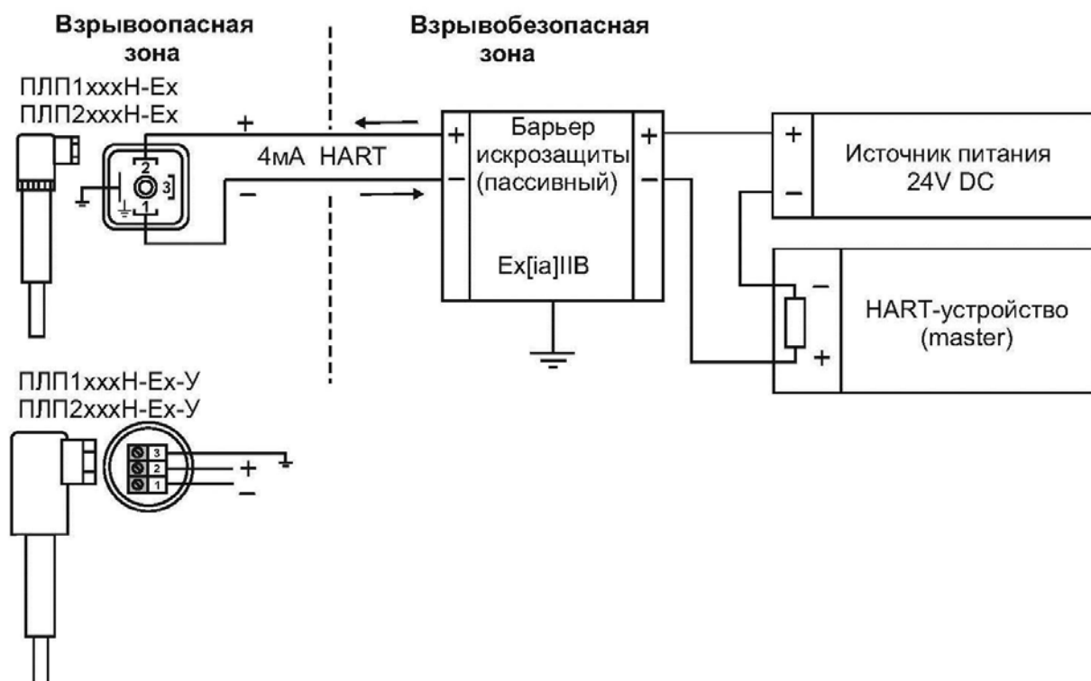
Рисунок 32 - Схема подключения уровнемеров ПЛП1xxxH-Ex(-У) и ПЛП2xxxH-Ex(-У) без гальванической развязки искробезопасных цепей
