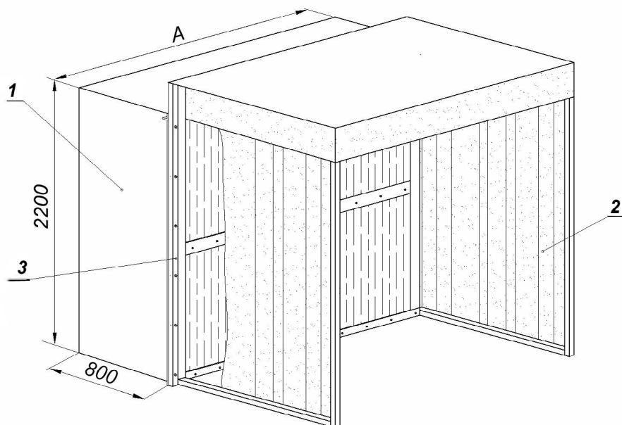
Рис.1. Схема покрасочной камеры
