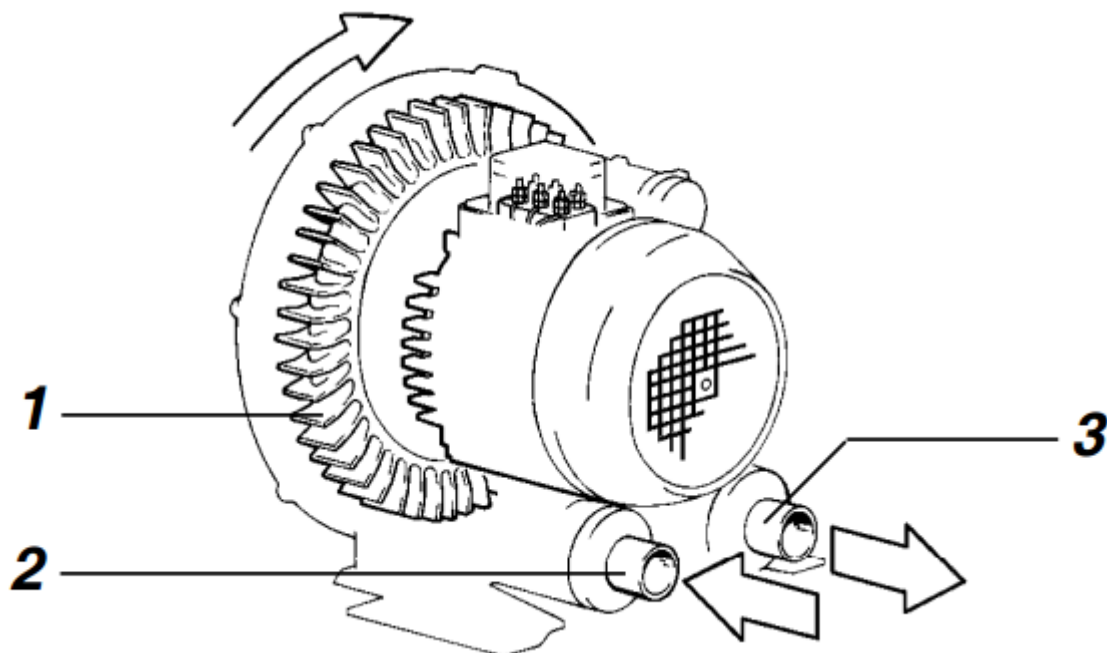
Рис. 1 – Общее устройство вихревой воздуховуки RB
