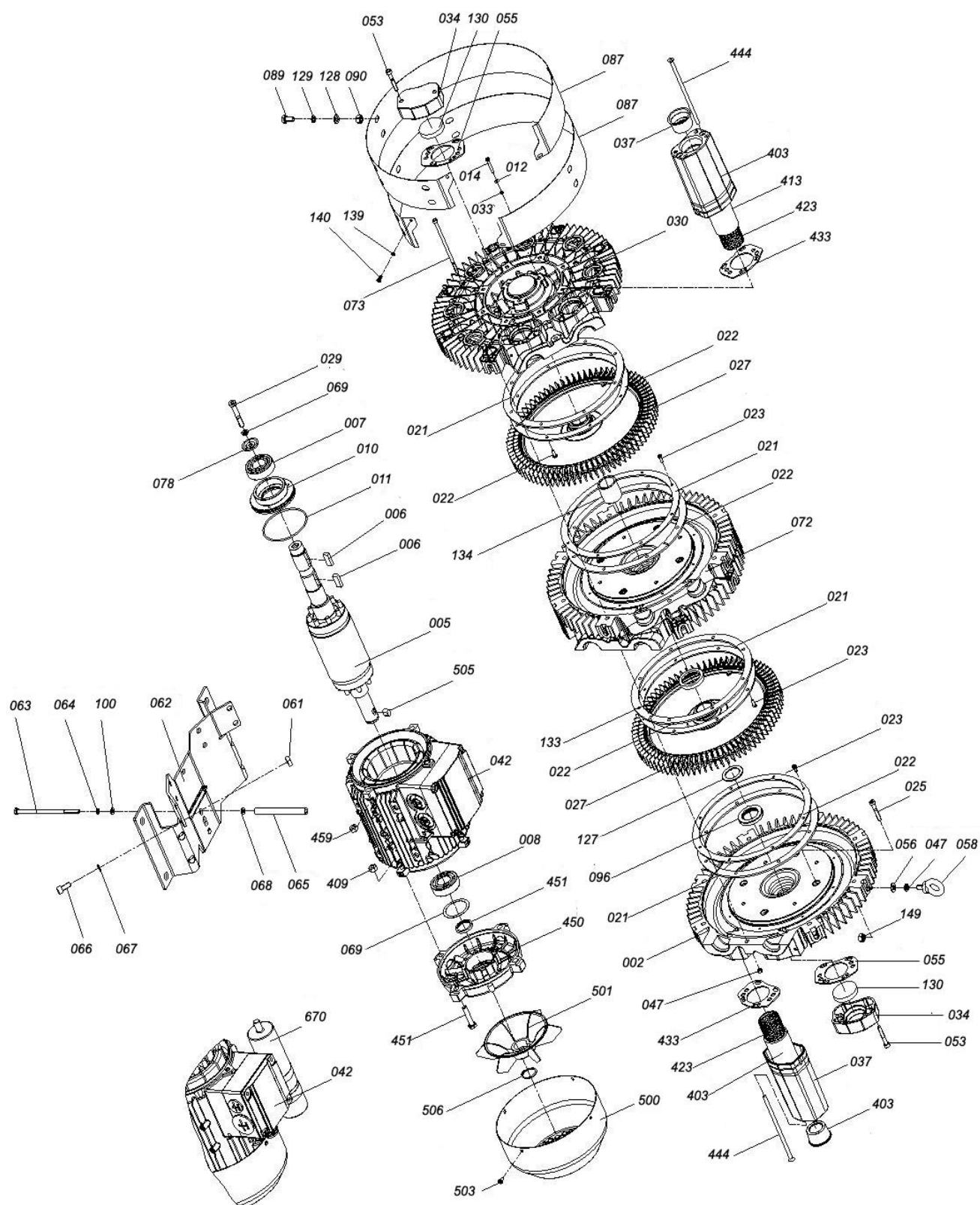
Рис. 5 – Детализовка двухступенчатых воздуховок 4RB
