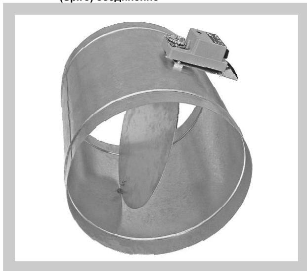
Рис. 1 Заслонка RKKM с сервоприводом, ниппельное (Spiro) соединение
