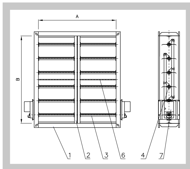
Рис. 5 Заслонка с управлением сервоприводом с разделяющей перегородкой (для A \geq 1300 ) с армирующим прутом (для B \geq 1200 )
