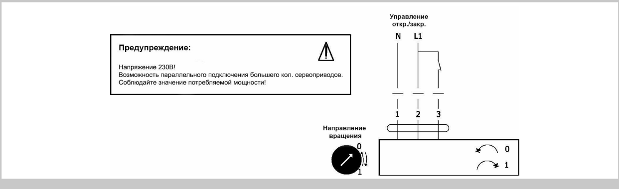
Рис. 8 Схема подключения сервопривода Belimo NM 24A, SM 24A и GM 24A
