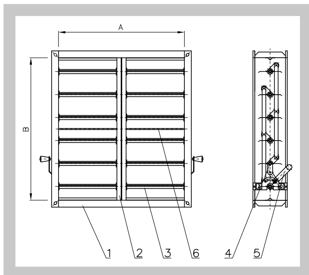
Рис. 4 Заслонка с ручным управлением с разделяющей перегородкой (для A \geq 1300 ) с армирующим прутом (для B \geq 1200 )
