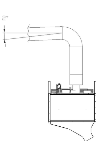
Горизонтальный дымоход через стену. Правильный монтаж
