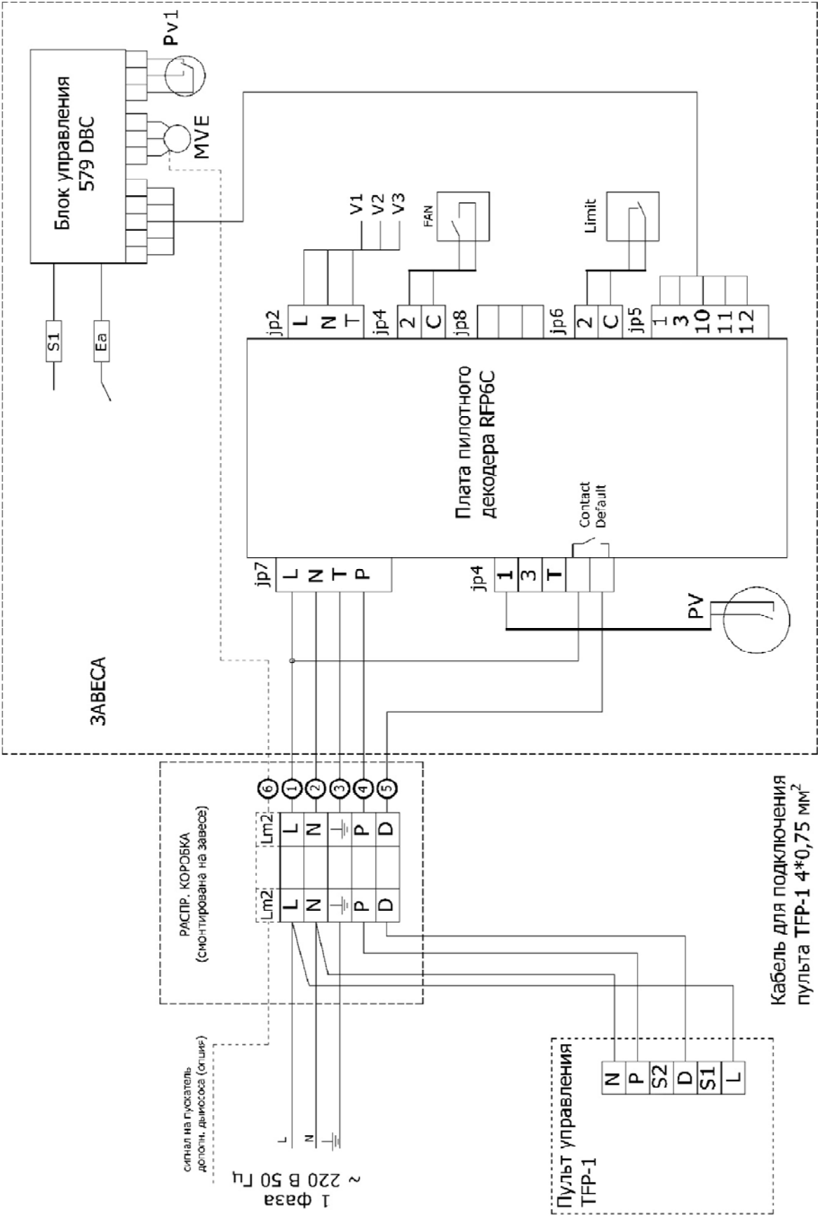
Рисунок 8.1.1 SA1 0035 ZT
