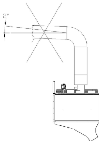
Горизонтальный дымоход через стену. Неправильный монтаж
