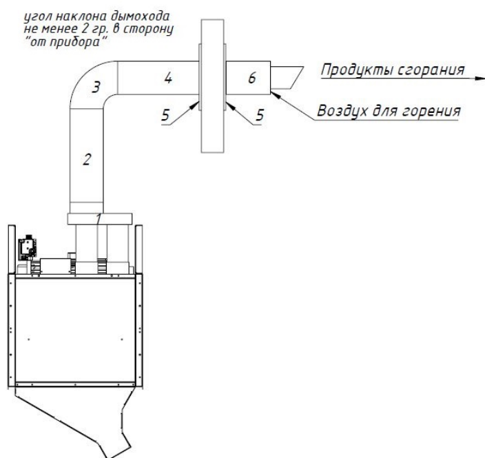
Рисунок 9.1.9 Горизонтальный коаксиальный дымоход. Горизонтальная установка завесы.
