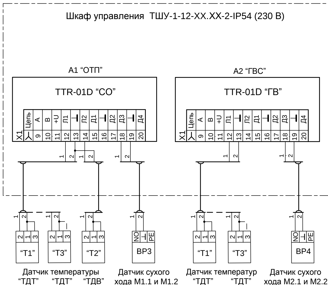
Рисунок Б.3 Схема подключения внешних датчиков
