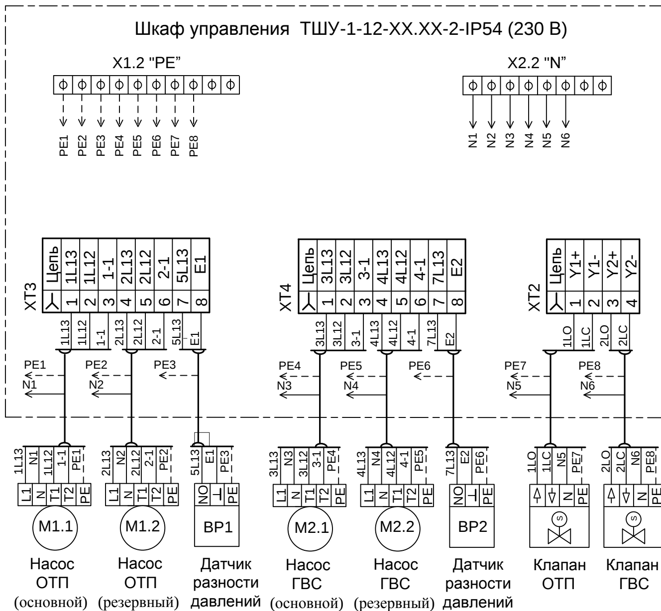
Рисунок Б.2 Схема подключения насосов и клапанов регулирующих
