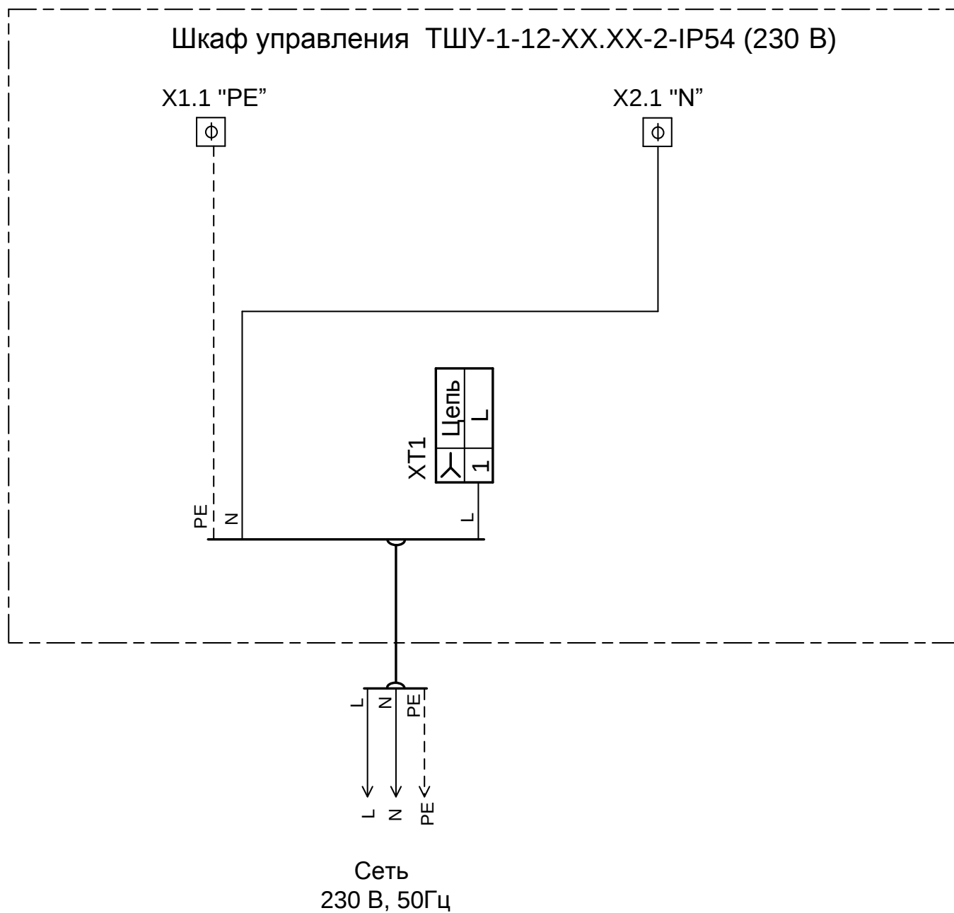
Рисунок Б.1 Схема подключения электропитания
