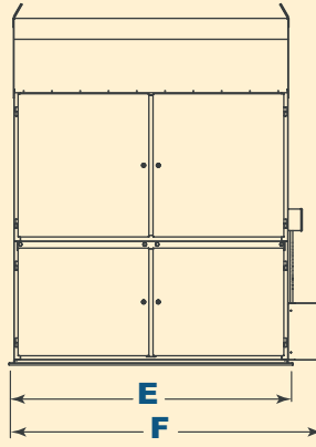
Front View UMA 450-750 (750 Shown)
