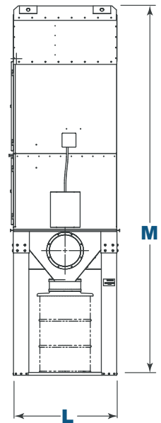
Right Side View UMA 450-750 (750 Shown)
