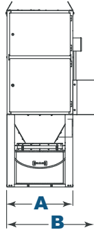
Front View UMA 70-250 (UMA 70 Shown)
