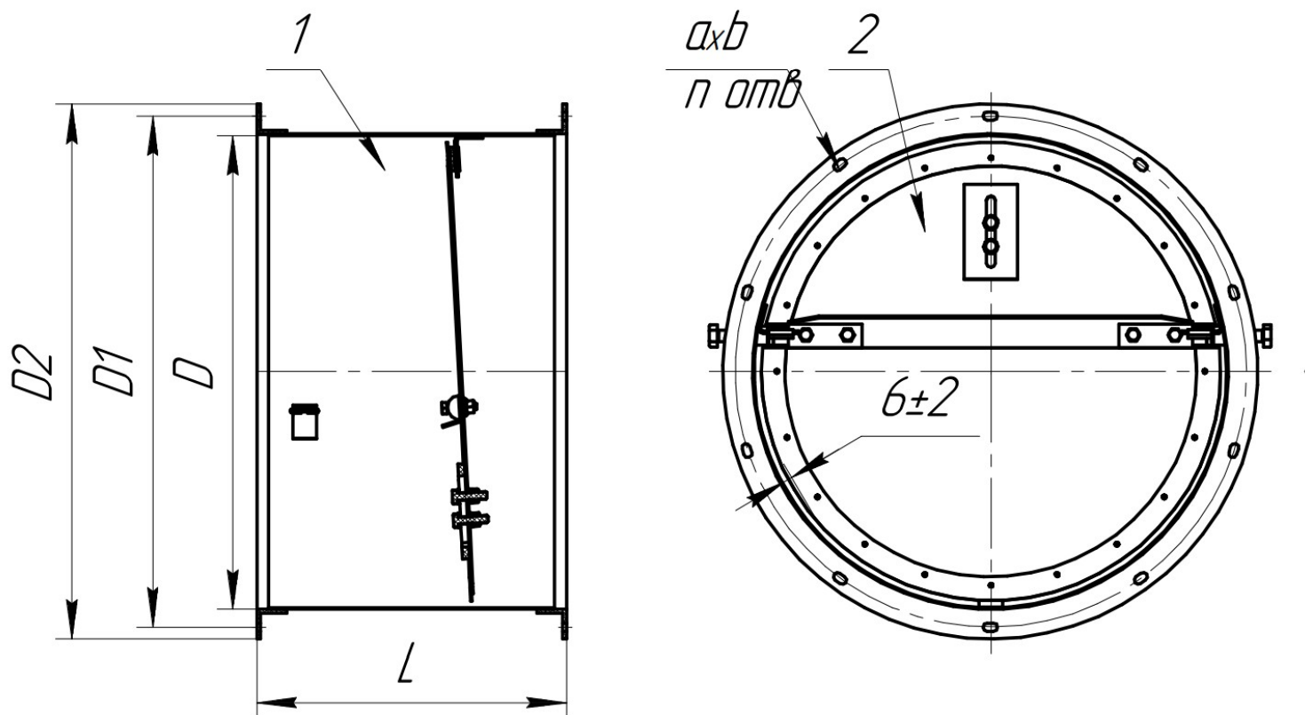
Рис. 4 1. Корпус, 2. Полотно
