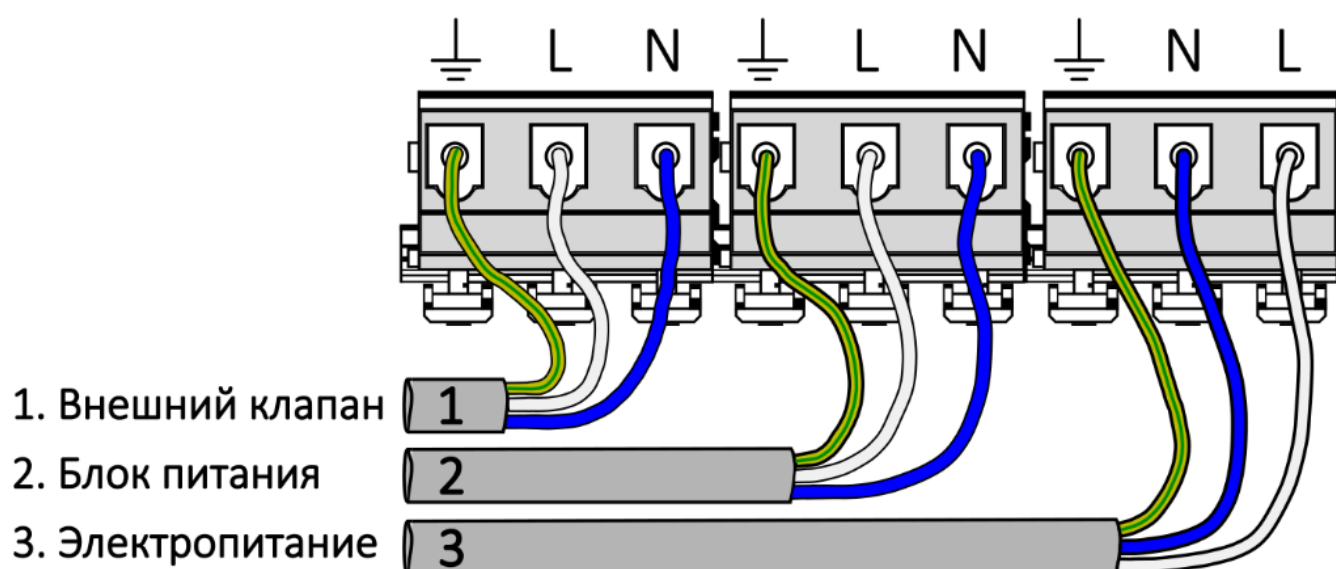
Рис. 4 Клеммная колодка
