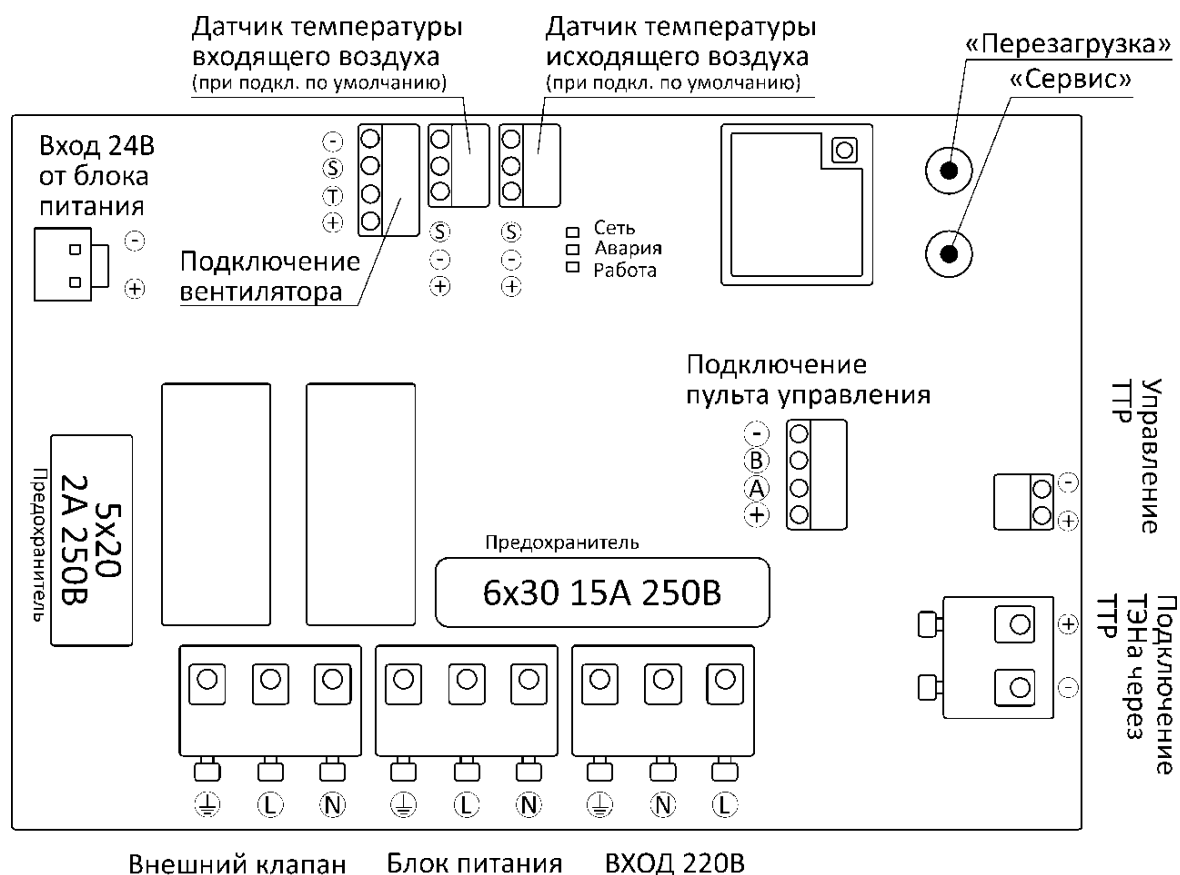
Рис. 9 Плата управления приточной установки
