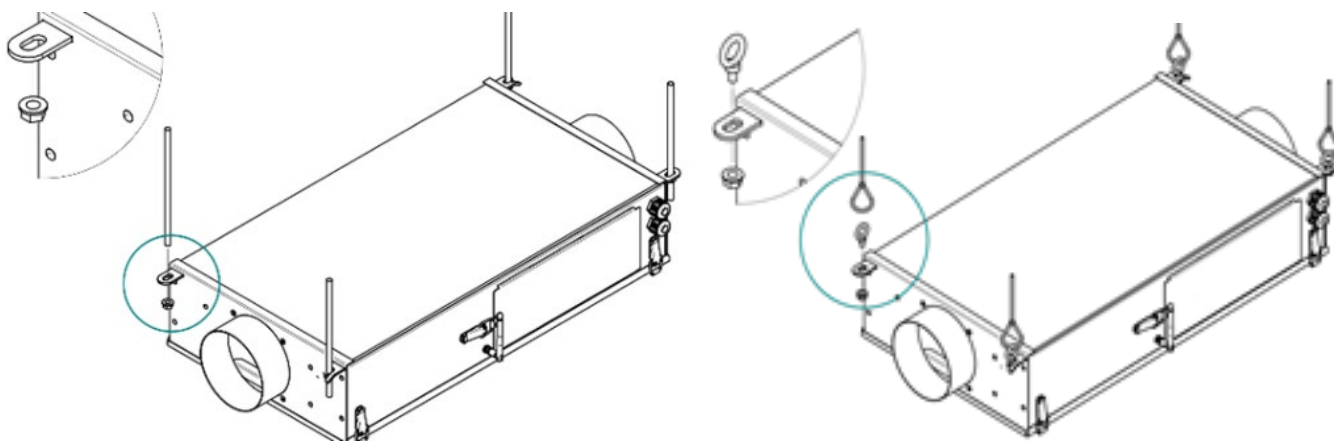
Рис. 3 Варианты монтажа вентиляционной установки
