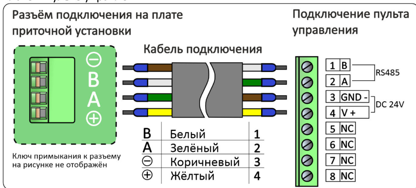
Рис. 5 Схема подключения пульта управления*
