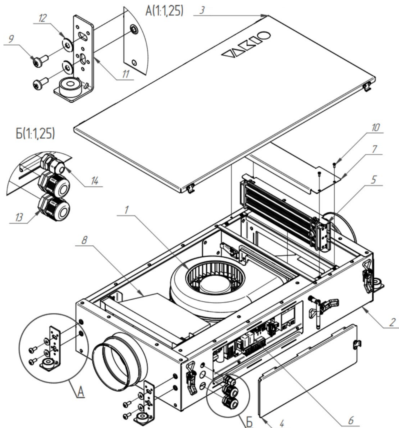
Рис. 1 Общий вид и внутреннее устройство приточной установки
