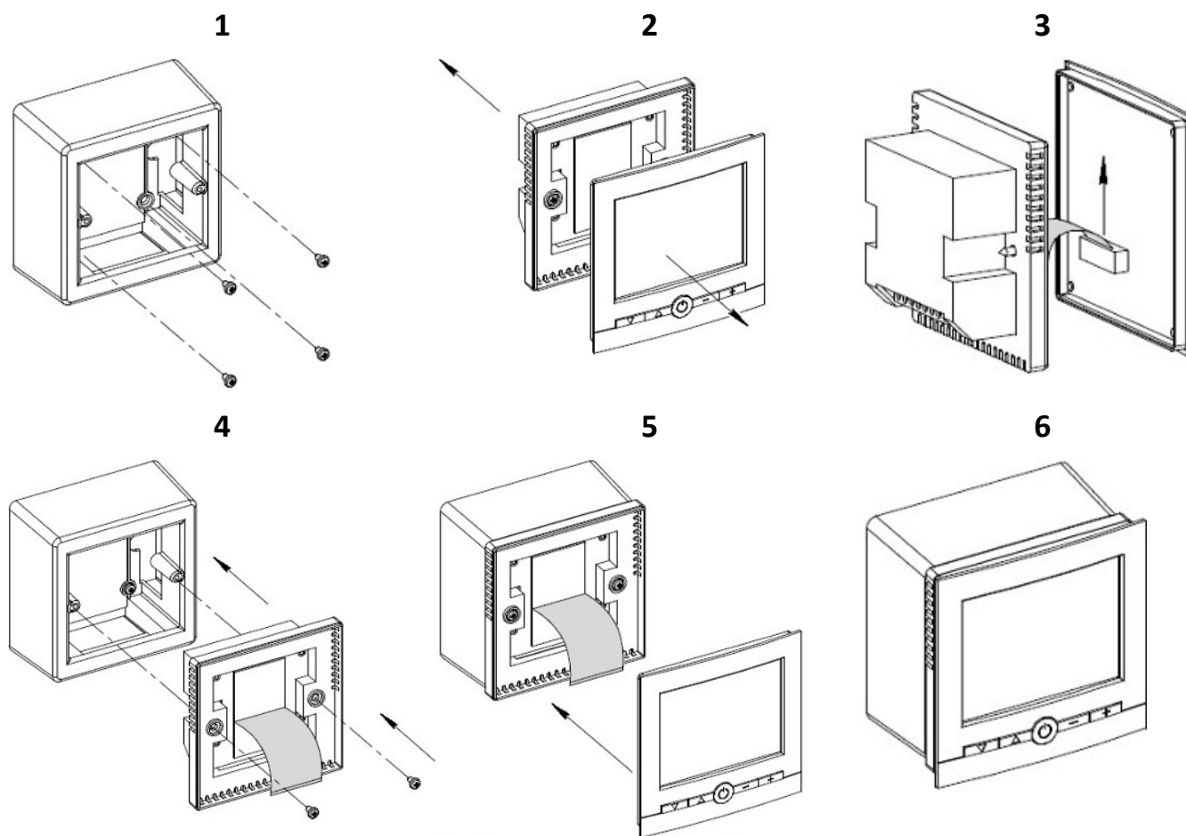
Рис. 6 Монтаж пульта управления
