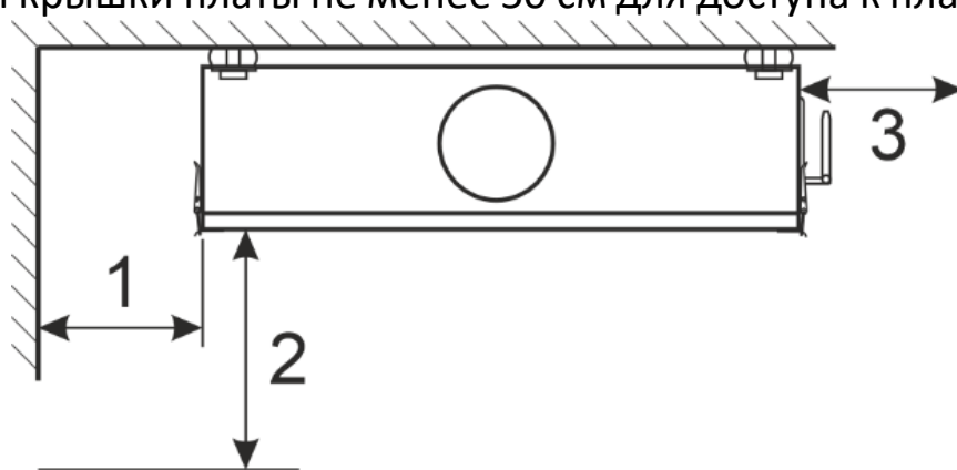
Рис. 2 Зона обслуживания. (Вариант монтажа на потолке).
