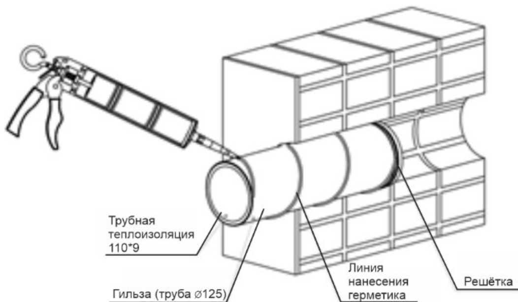
Рис. 4 Вариант установки гильзы с нанесением герметика
