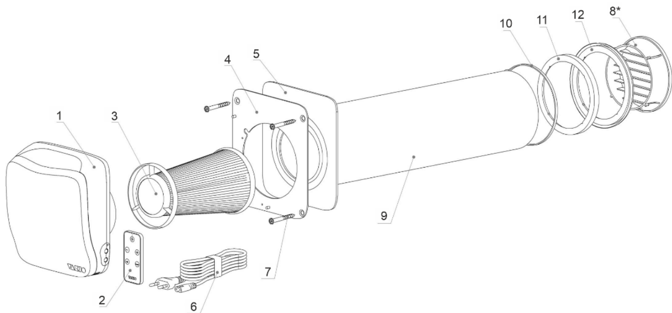
Рис. 2 Состав комплекта поставки. *Вариант с пластиковой решеткой.
