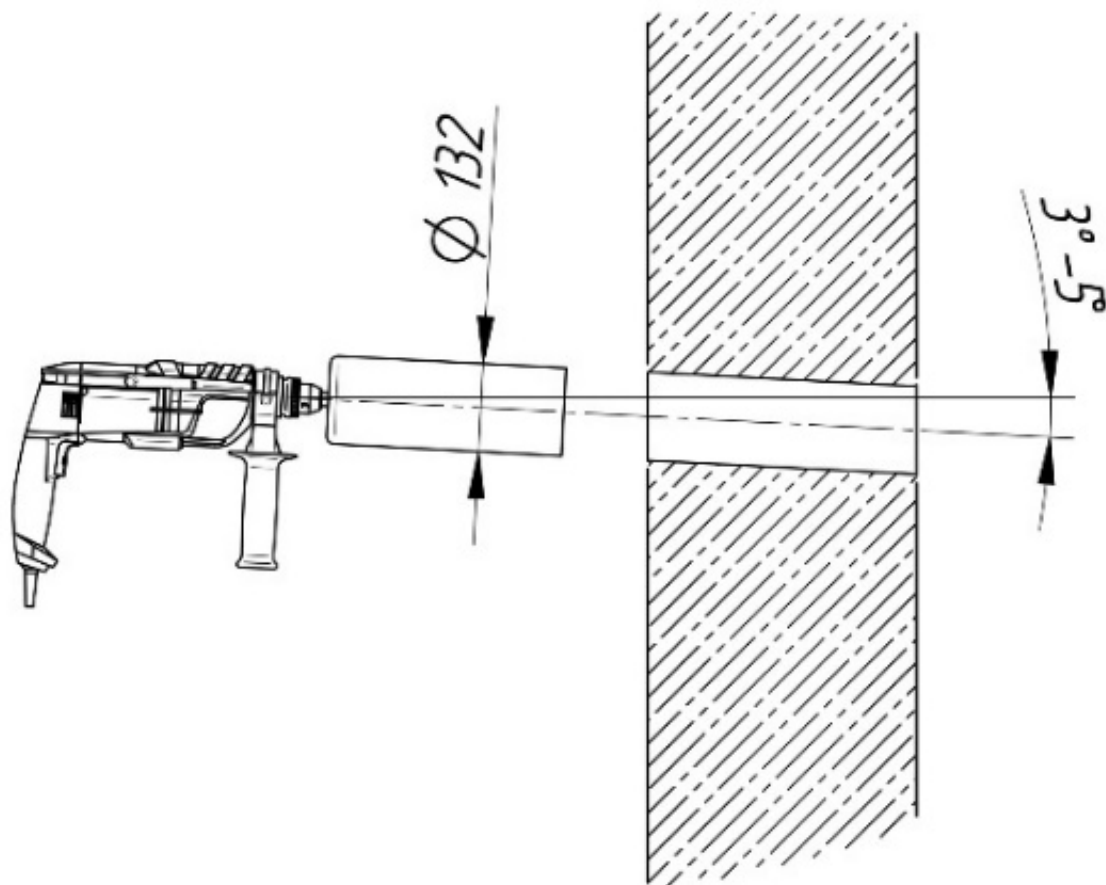
Рис. 3 Бурение отверстия
