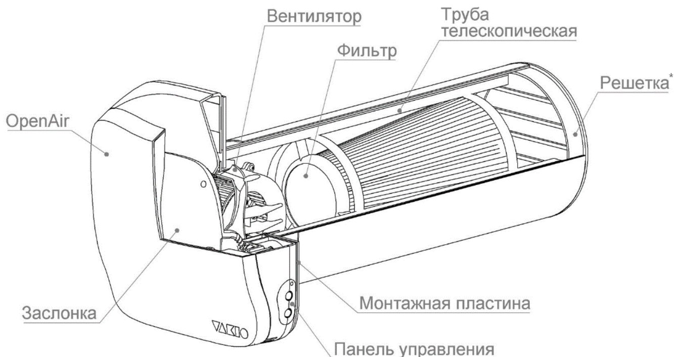
Рис. 1 Общий вид прибора. *Вариант с металлической решёткой.
