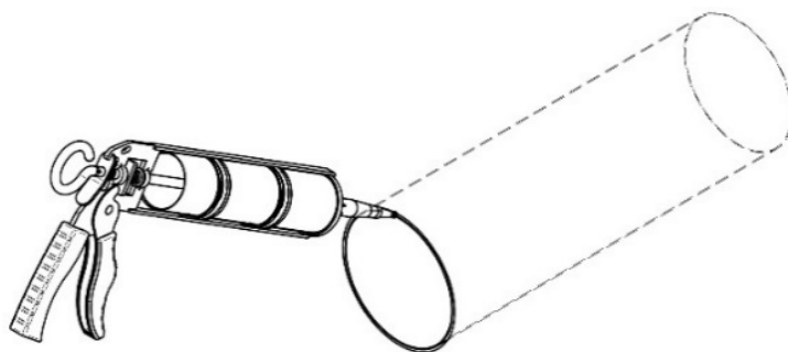
Рис. 5 Герметизация трубы канала
