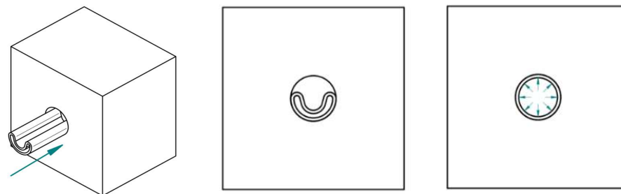
Рис. 6. Установка теплоизоляции в канал трубы.
