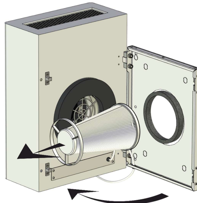
Рис. 10. Замена фильтра.
