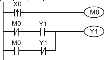
Пример 9: триггерная схема
