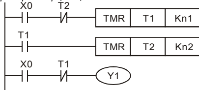
Пример 8: мерцающая схема
