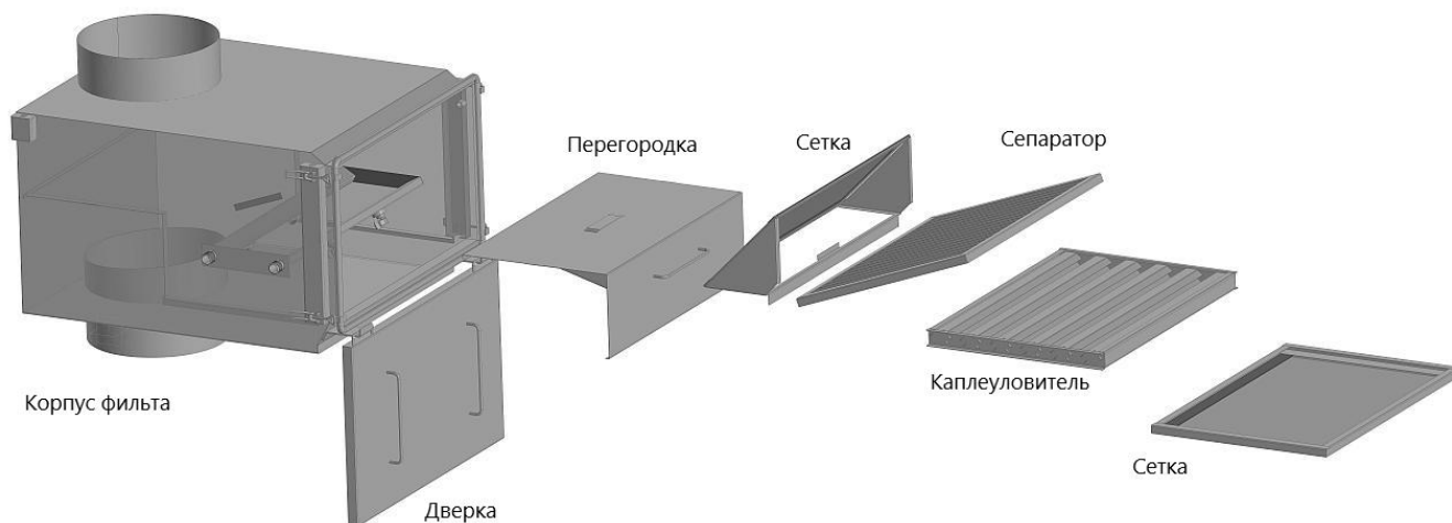
Рис. 3 Схема последовательности разбора, для очистки фильтра-искрогасителя:
