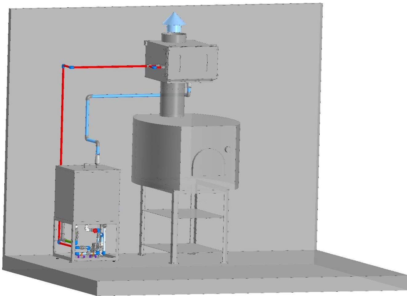
Рис. 1 Схема размещения фильтра ГФ
