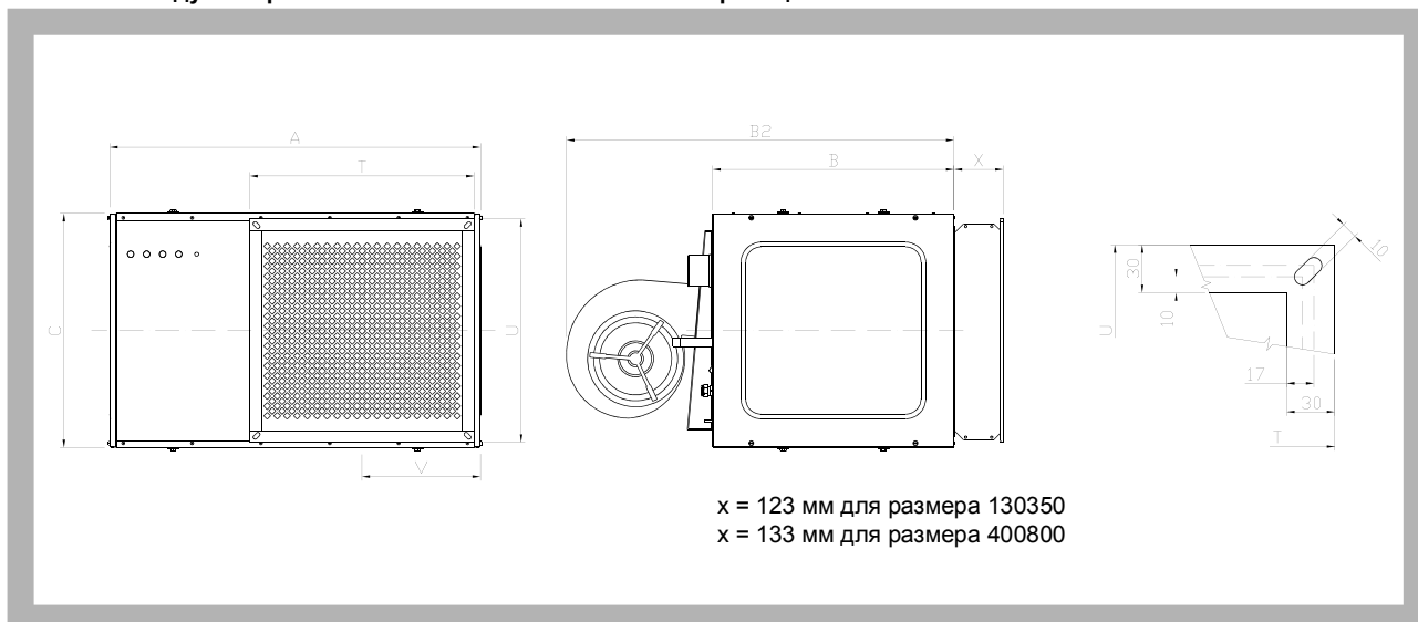
Рис. 9. Воздухонагреватель MONZUN CV - исполнение с фланцем
