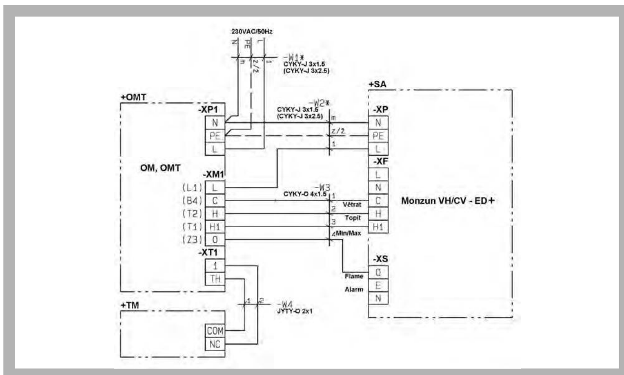
Рис. 40. Схема подключения агрегата MONZUN с шкафом управления ОМ, ОМТ для VH 130ED+ 700ED+ и CV 130ED+ 800ED+ с однофазным вентилятором.
