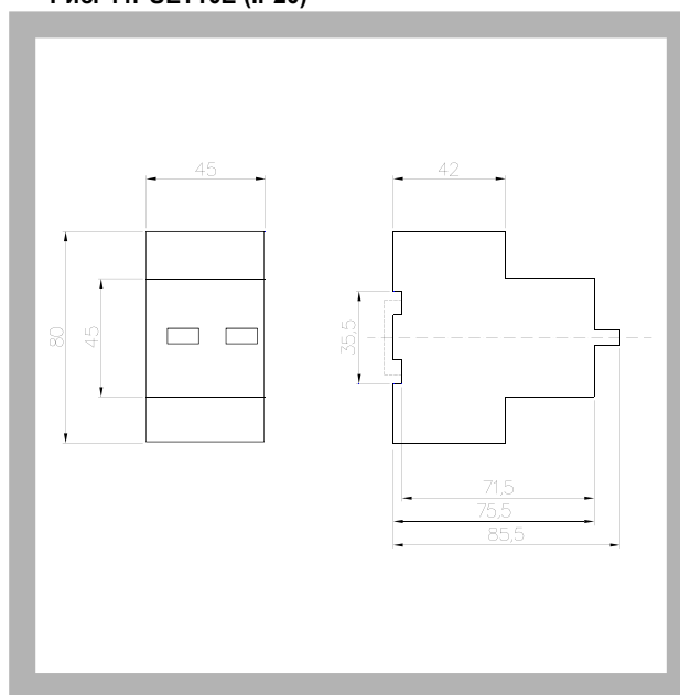
Рис. 44. SET10E (IP20)
