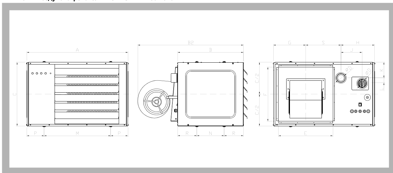
Рис. 7. Воздухонагреватель MONZUN CV 130 - 520
