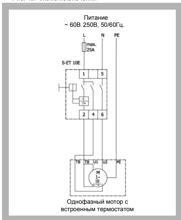
Рис. 45. Схема подключения
