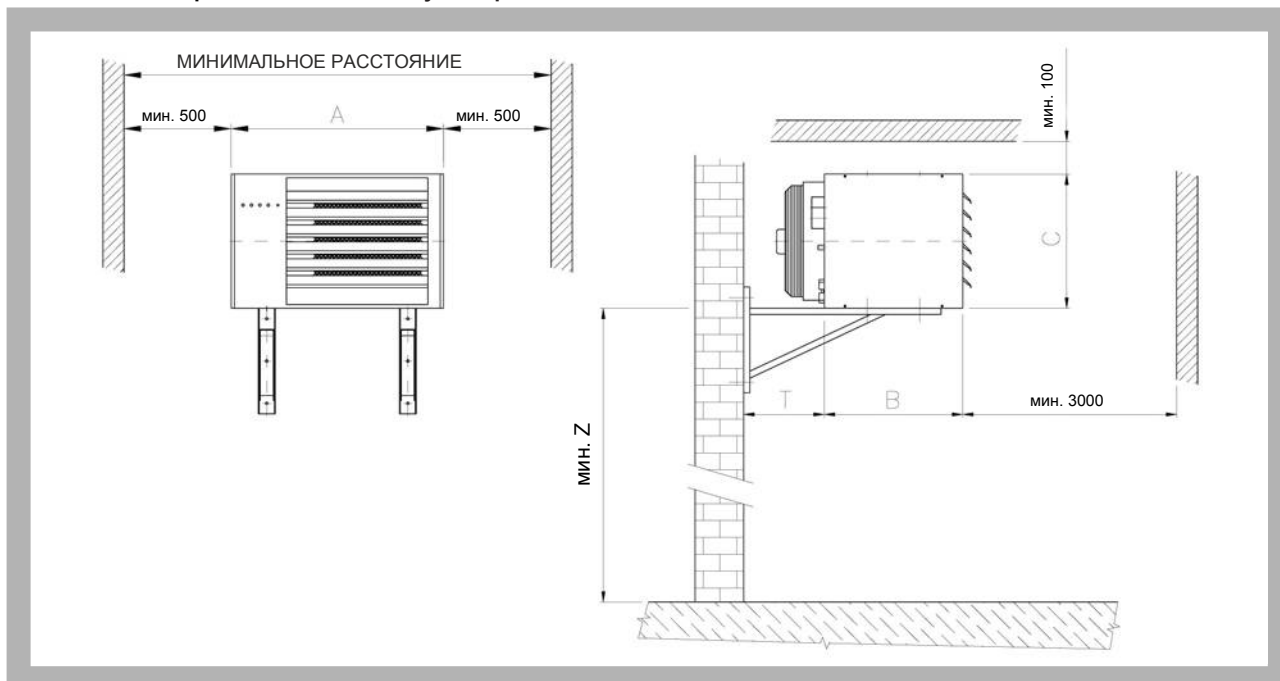
Табл. 6.1.1. Воздухонагреватели MONZUN VH/CV - монтажные размеры
