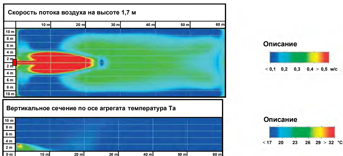
Рис. 19. MONZUN 450. Максимальный расход воздуха, жалюзи развернуты на 45°, температура среды 18°C
