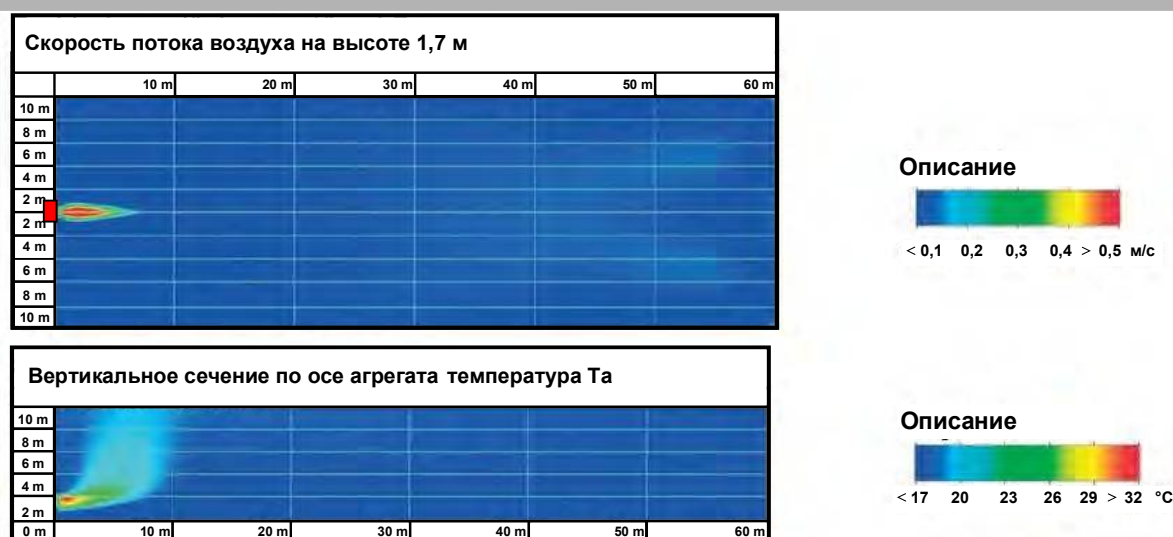
Рис. 13. Воздухонагреватель MONZUN 130. Макс. расход воздуха, положение жалюзи - 45°, температура окружающей среды 18°C
