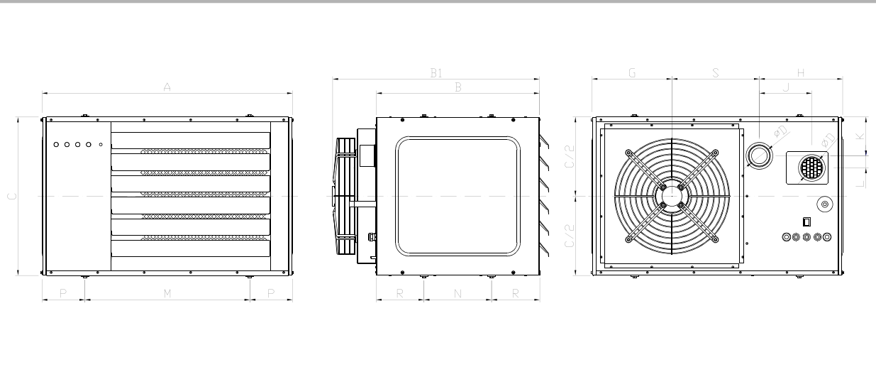
Рис. 6. Воздухонагреватель MONZUN VH 600 - 700
