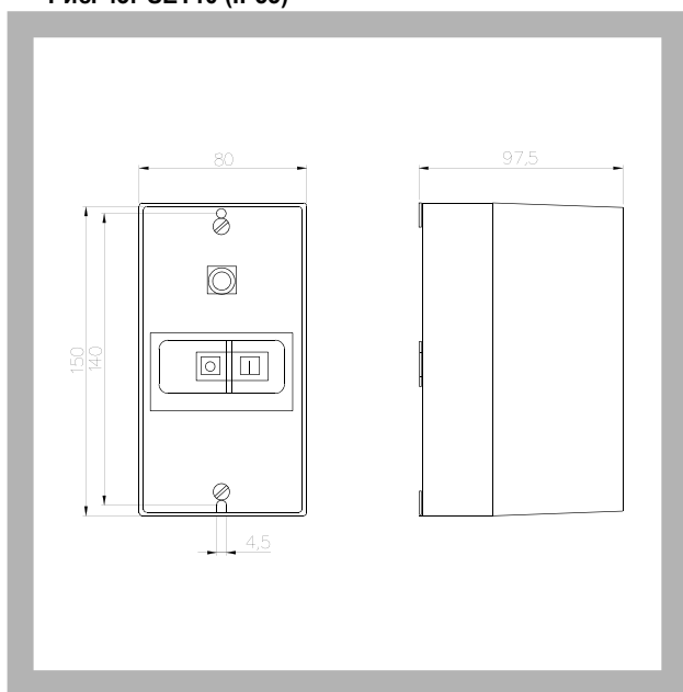
Рис. 43. SET10 (IP55)
