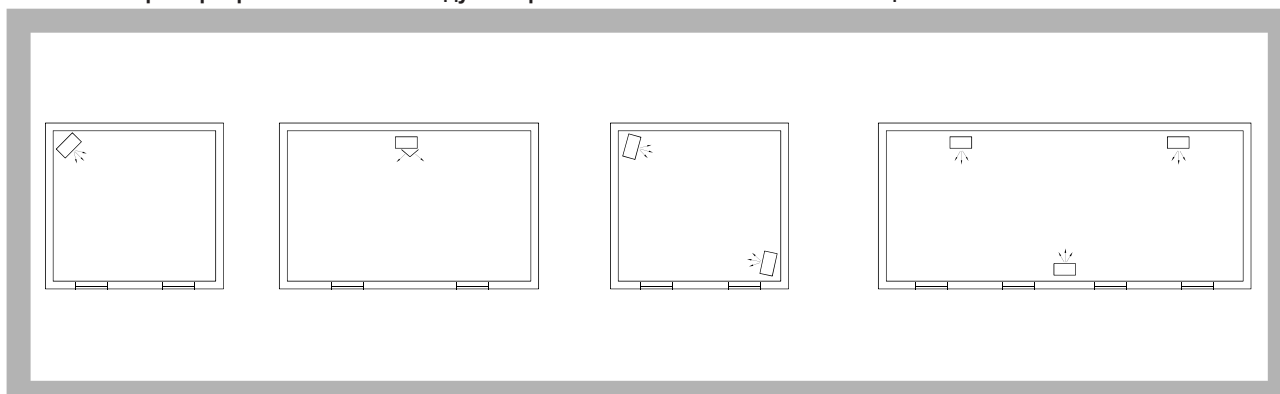
Рис. 12. Примеры расположения воздухонагревателей в отапливаемом помещении
