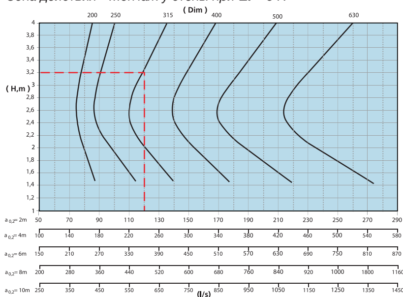
Диаграмма 3. Зона действия - Монтаж у стены при \Delta t = 3 \text{ K}
