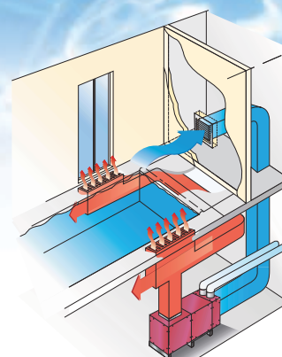
Установка расположена в подвальном помещении, подача воздуха снизу. Установлен модуль приточно-вытяжной вентиляции.
