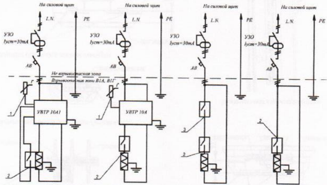
Рис1. Для нагревателей ВНУ-1600Б ВНУ-2000Б
