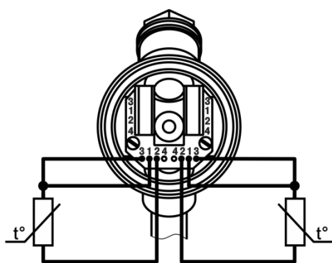
Рисунок Д.8 – Трехпроводная схема подключения проводов к клеммам коммутационной головки с двумя ЧЭ
