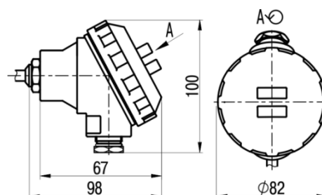
Рисунок В.3 – Увеличенная металлическая коммутационная головка
