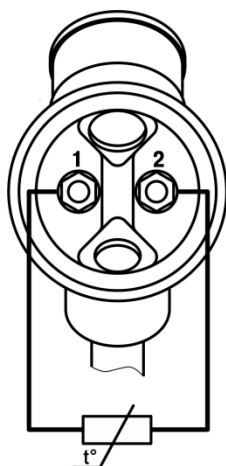
Рисунок Д.1 – Двухпроводная схема подключения проводов к клеммам пластмассовой коммутационной головки с одним ЧЭ
