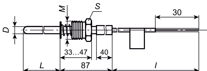
Рисунок А.6 – Конструктивные исполнения 124, 134 и 144
