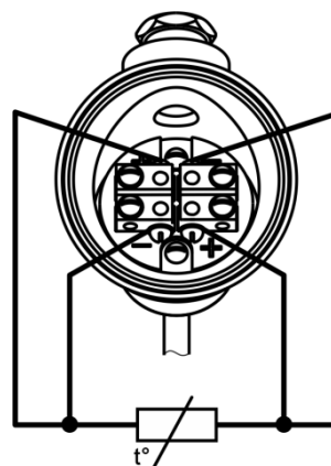
Рисунок Д.6 – Четырехпроводная схема подключения проводов к клеммам металлической коммутационной головки с одним ЧЭ
