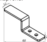
СКОБА
