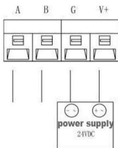
Выход RS485
