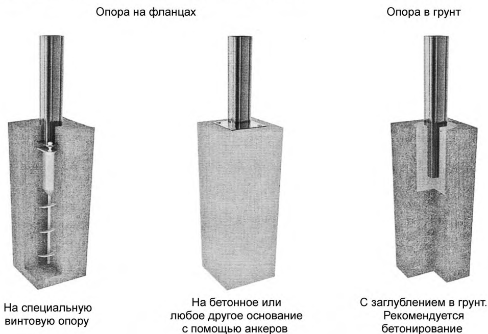
Рисунок 1 — Основные виды установки опор
