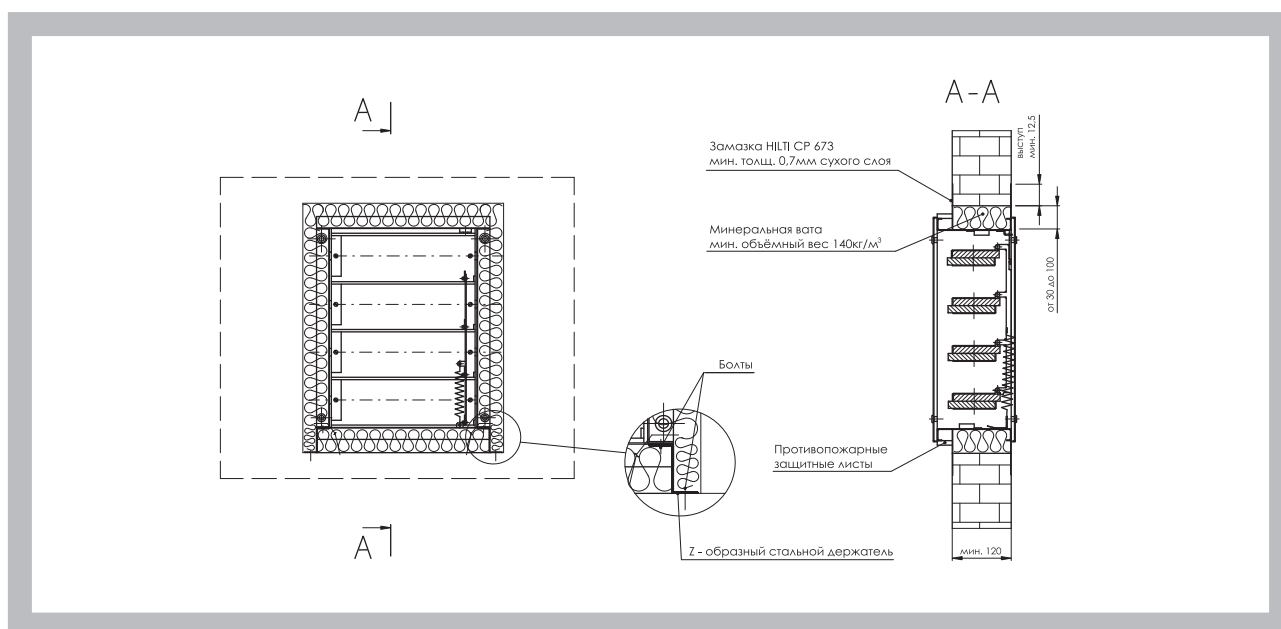
Рис. 10 Способ монтажа в жестких стеновых конструкциях - минвата, замазка HILTI CP 673
