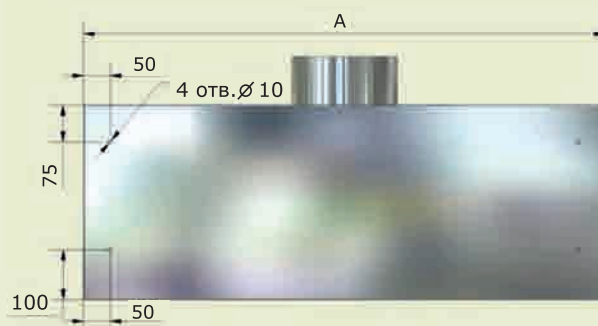
МВО - (А) МС (МСВ) - 08М х (В) Расположение отверстий для подвески к потолку. Вид сверху.
