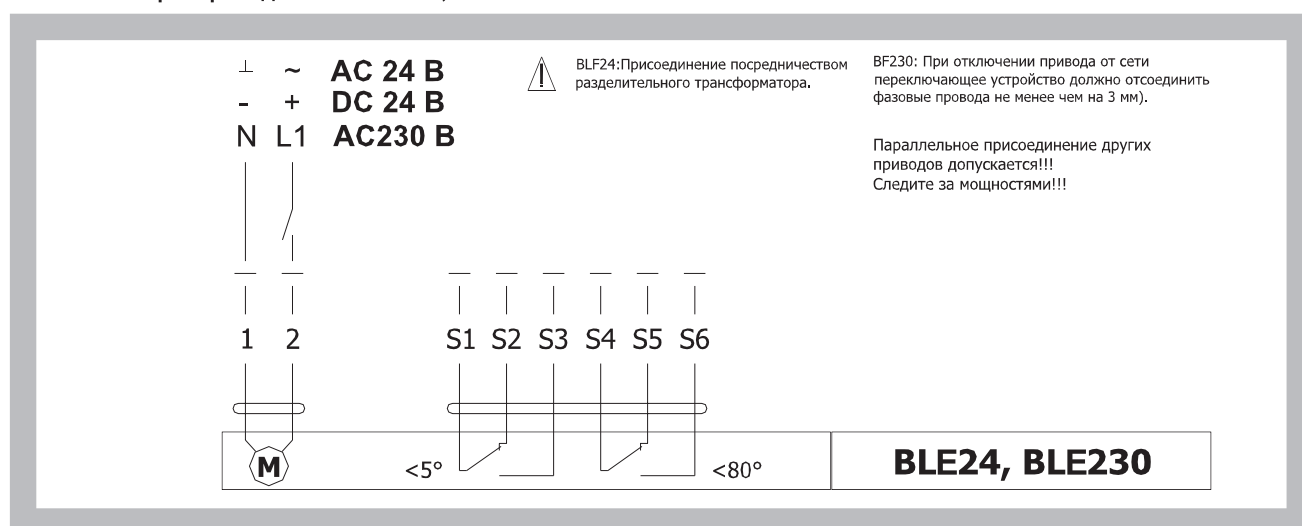
Рис. 18 Сервопривод BELIMO BLE 24, BLE 230
