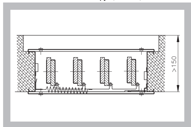
Рис. 17 Потолочная конструкция толщ. < 150 мм
