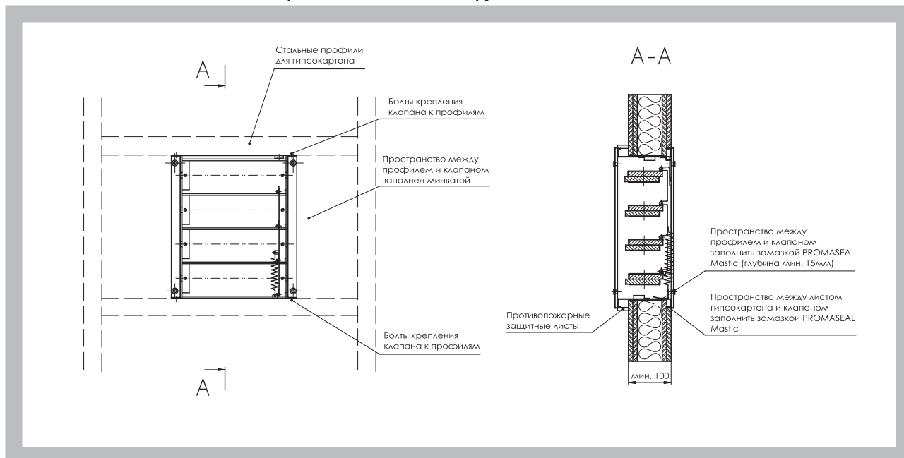
Рис. 11 Способ монтажа в гипсокартонные стеновые конструкции - замазка PROMASEAL-Mastic
