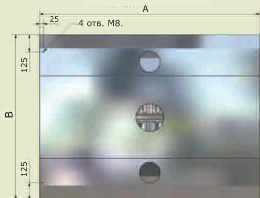
МВО - (А) МС (МСВ) - 07 х (В) Расположение отверстий для подвески к потолку. Вид сверху.
