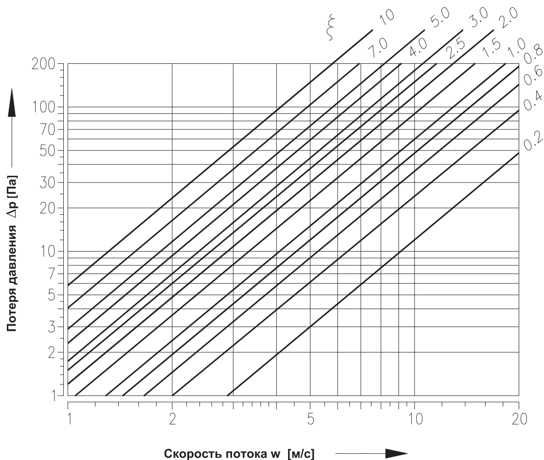
Рис. 24. Диаграмма потерь давления
