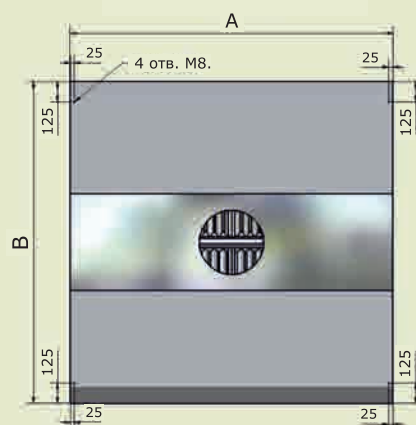
МВО - (А) МСВ - 07С х (В) Расположение отверстий для подвески к потолку. Вид сверху.
