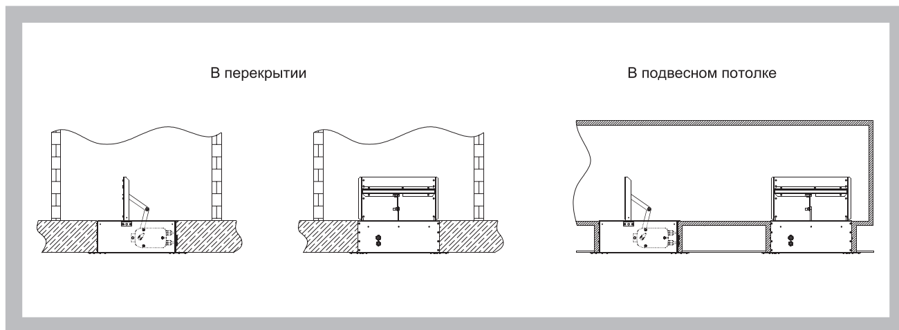
Рис. 10 Примеры установки клапанов «стенового» исполнения в горизонтальной плоскости
