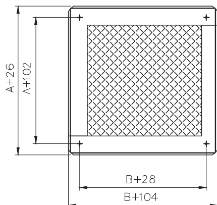
Рис. 22 Решетка
