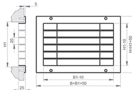
Нерегулируемая решетка РВА9
