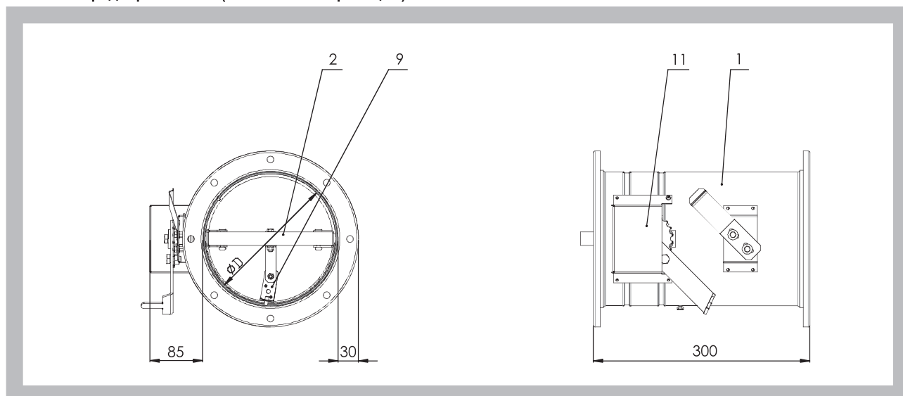
Рис. 6. Круглый противопожарный клапан исполнение с ручным управлением и тепловым плавким предохранителем (исполнение с фланцем)
