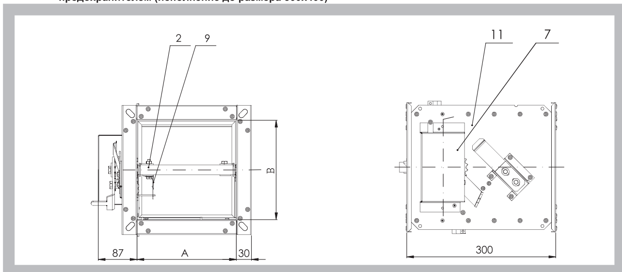
Рис. 3. Прямоугольный противопожарный клапан исполнение с ручным управлением и тепловым плавким предохранителем (исполнение от размера 500x400мм)
