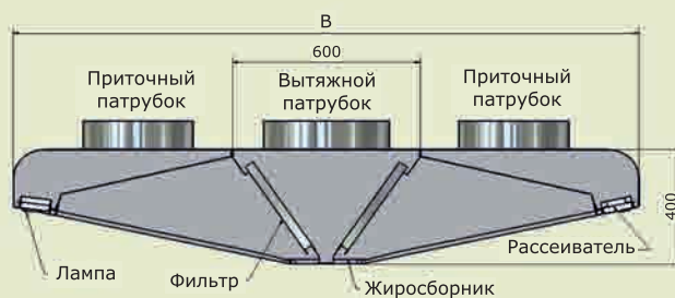
МВО - (А) МС -07СО x (В) Устройство
