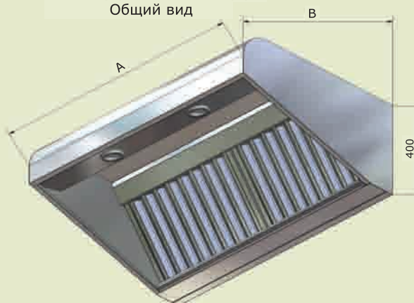
МВО - (А) МСВ - 08М х (В) Общий вид
