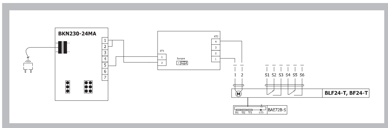
Рис. 42. Подключение с сервоприводом BF 24-T (BLF 24-T), оптической дымовой сигнализацией MHG 231 и блоком питания BKN 230-24-MA (напряжение оборудования AC 230B)
