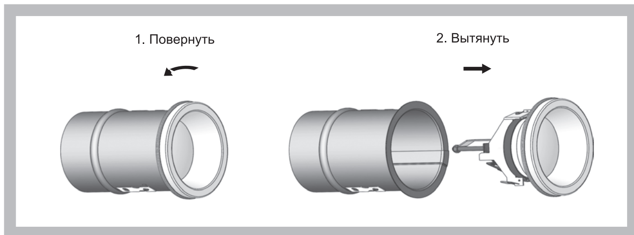
Рис. 7 Схема демонтажа противопожарного клапана
