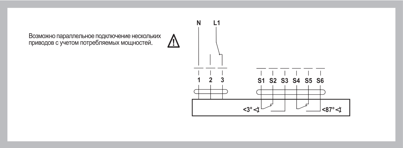
Рис. 18. Монтажная схема подключения сервопривода BELIMO BLE 24, BLE 230
