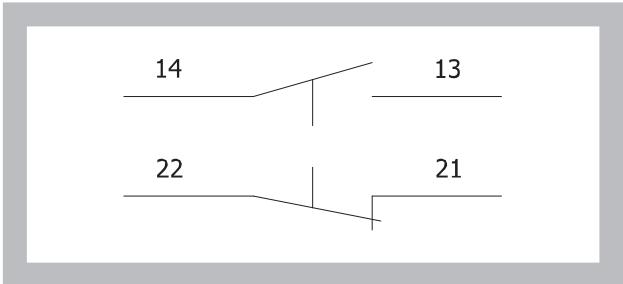
Рис. 25. Концевой выключатель XCKN2118G-115
