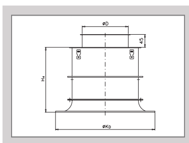
вертикальное присоединение VASM... / S
