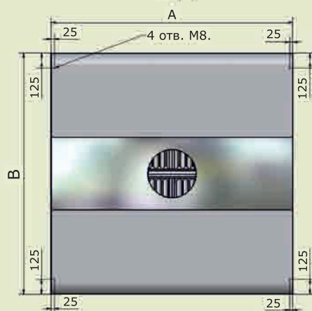
МВО - (А) МСВ - 07СО х (В) Расположение отверстий для подвески к потолку. Вид сверху.
