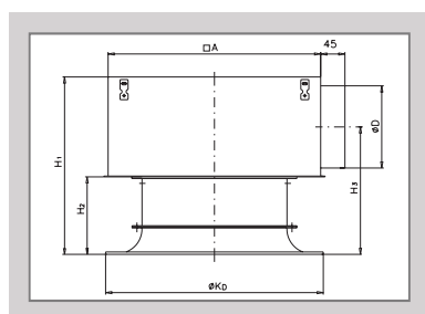
горизонтальное присоединение VASM... / V
