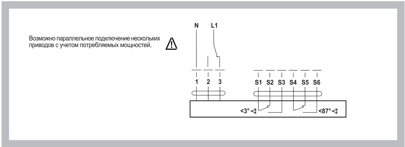
Рис. 20 Монтажная схема подключения сервопривода BELIMO BE 24, BE 230
