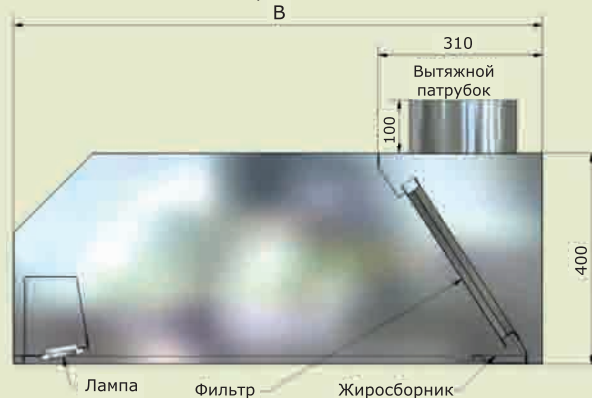
МВО - (А) МСВ - 06 x (В) Устройство
