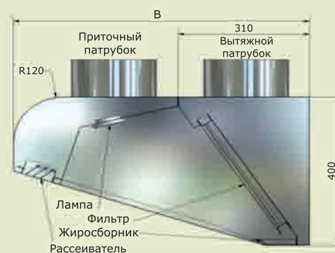
МВО - (А) МС -08М x (В) Устройство
