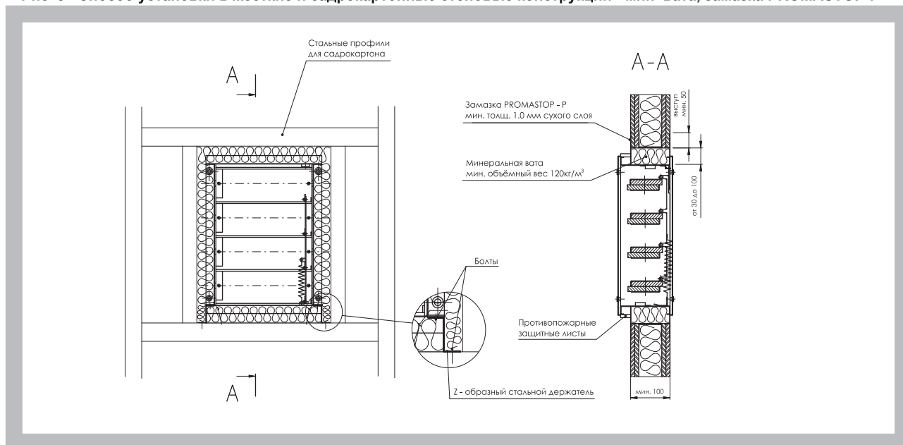
Рис. 9 Способ установки в жесткие и садрокартонные стеновые конструкции - мин. вата, замазка PROMASTOP-P
