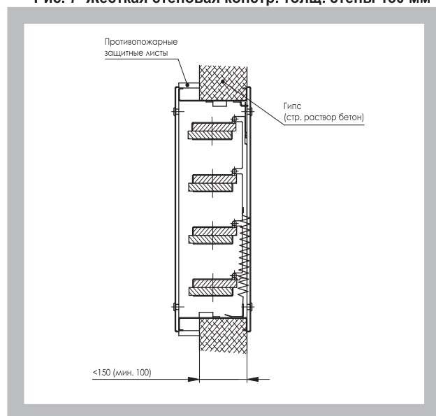
Рис. 7 Жесткая стеновая констр. толщ. стены 150 мм
