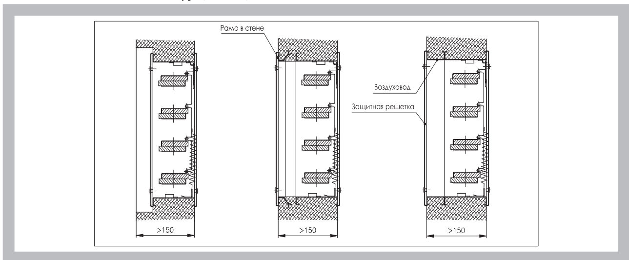
Рис. 18 Жесткая стеновая конструкция толщ. > 150 мм
