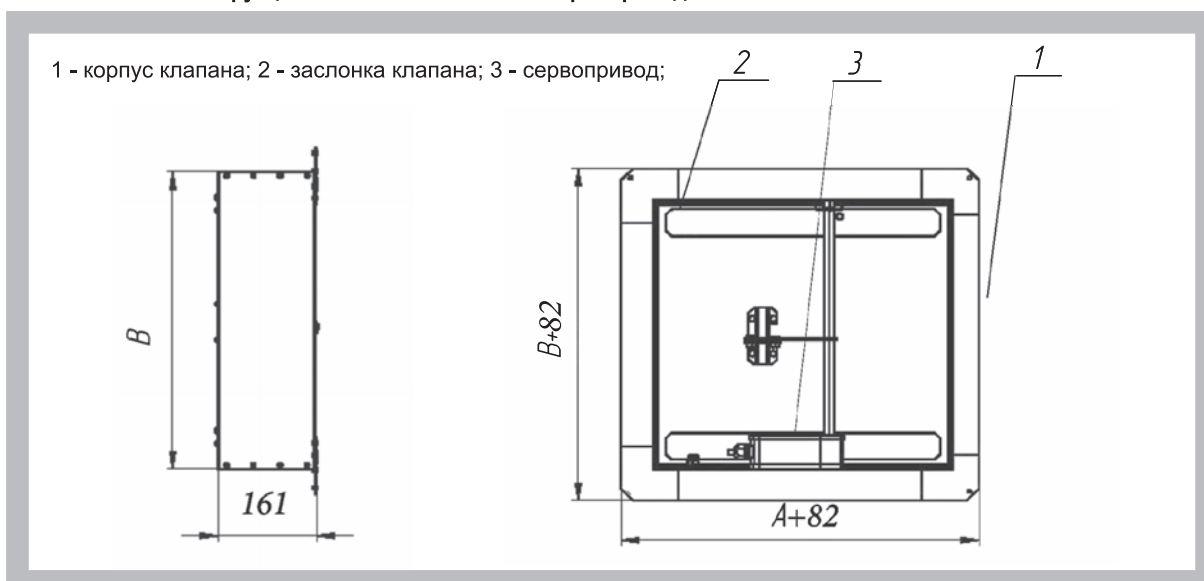
Рис. 3.3. Схема конструкции клапана ОКМ EI-90 с сервоприводом Belimo
