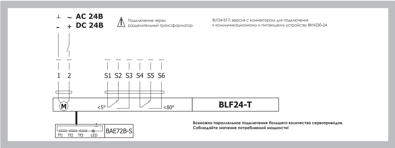
Рис. 22 Сервопривод BELIMO BLF 24-T
