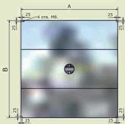
МВО - (А) МСВ - 07М х (В) Расположение отверстий для подвески к потолку. Вид сверху.
