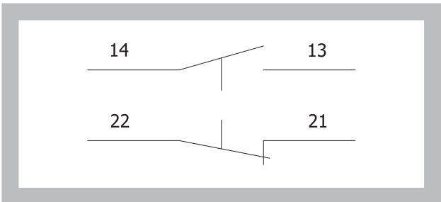
Рис. 20 Концевой выключатель XCKN2118G-11
