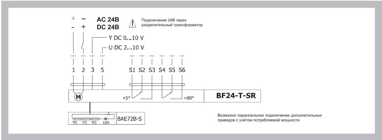
Рис. 34. Сервопривод BELIMO BF 24-T-SR
