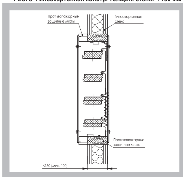
Рис. 8 Гипсокартонная констр. толщин. стены < 150 мм
