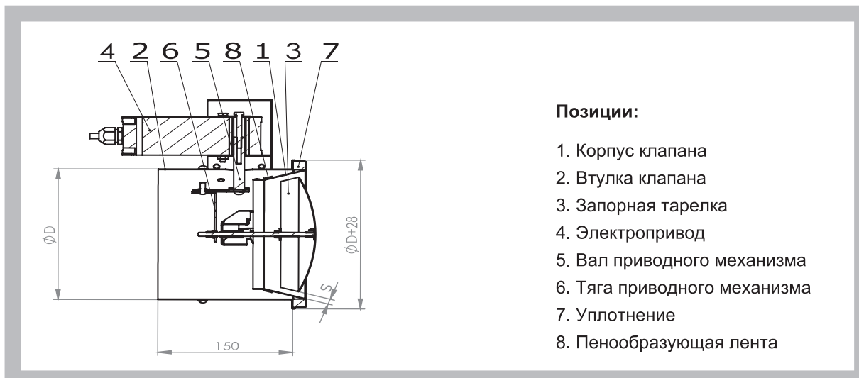
Рис. 3 Устройство клапана противопожарного PVM - E90 с электроприводом Belimo (установка электропривода параллельно оси клапана) – В – вертикальная установка
