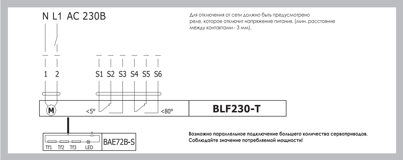
Рис. 23 Сервопривод BELIMO BLF 230-T
