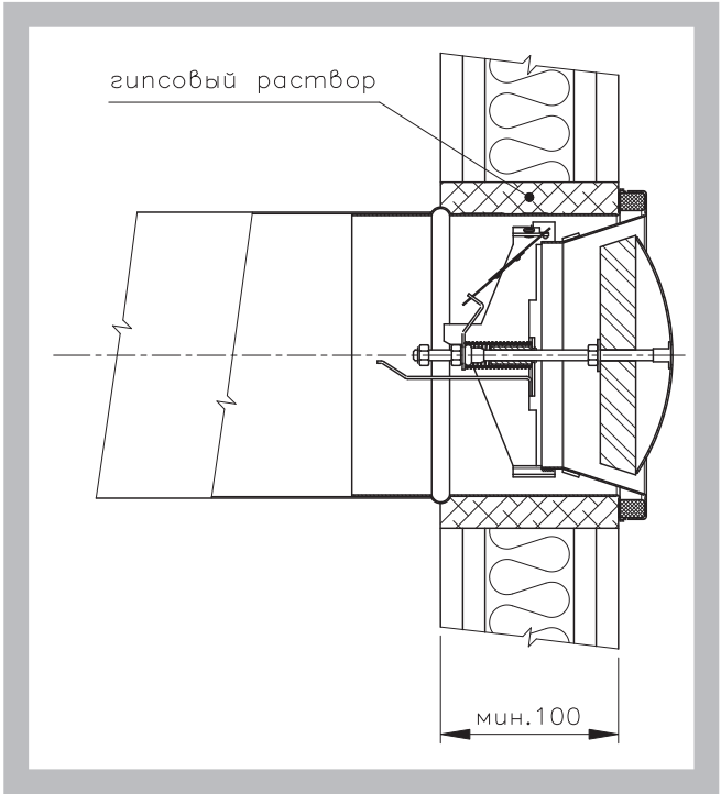
Рис. 6 С присоединением к воздуховоду
