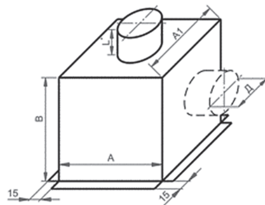
УП2-Т (штриховой линией показан УП2-Б)
