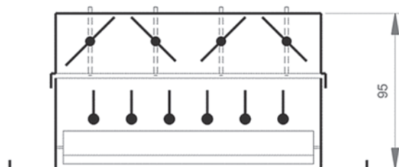
Регулируемая вентиляционная решетка РВС2-А-Б1, РВА2-А-Б1 (с клапаном Б1)
