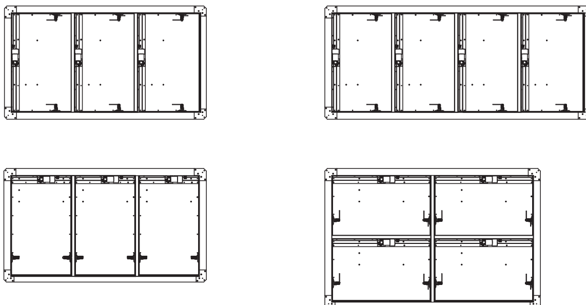
Рис. 7 Схема конструкции клапана ОКМ - 90 кассетного исполнения
