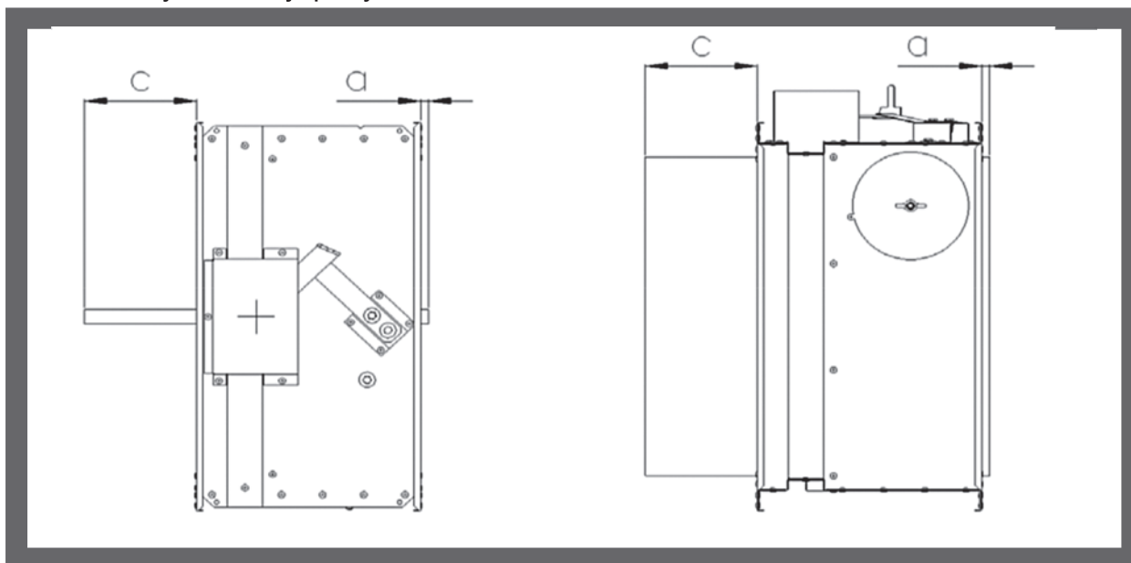
Рис. 13. Выступ заслонки у круглого клапана с фланцем
