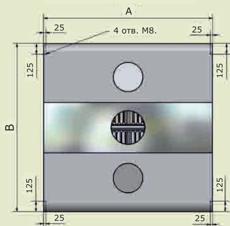
МВО - (А) МС - 07СО х (В) Расположение отверстий для подвески к потолку. Вид сверху.
