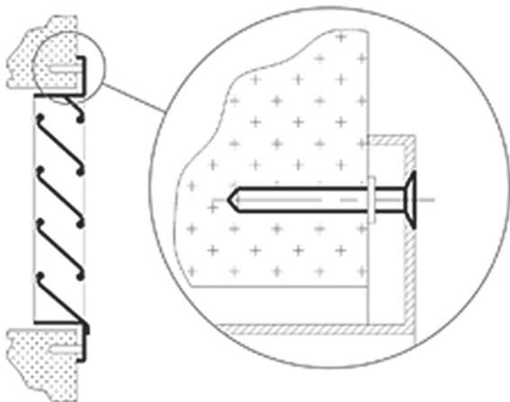
Монтаж РВС4, РВА4
