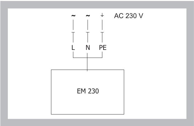
Рис. 13 Электромагнит EM230
