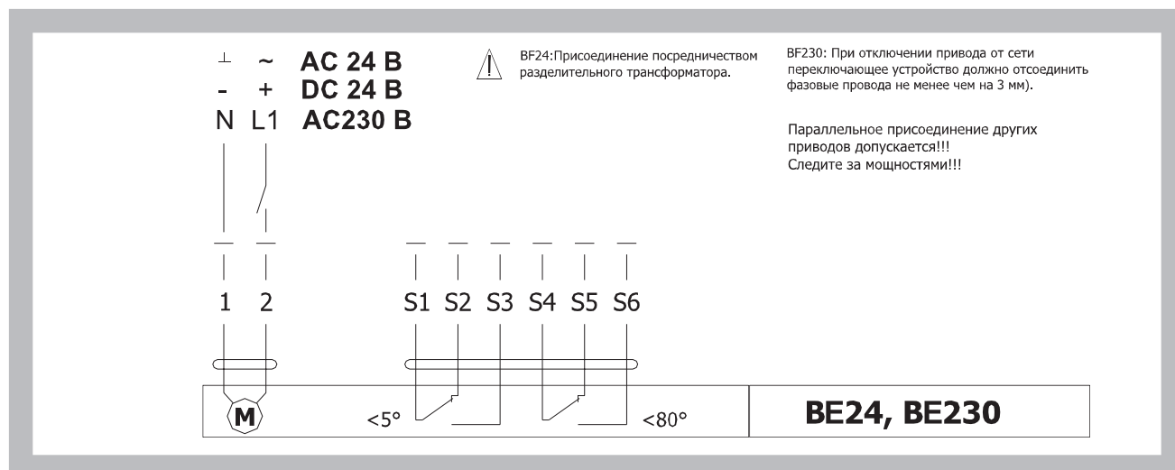
Рис. 20 Сервопривод BELIMO BE 24, BE 230
