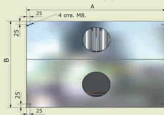
МВО - (А) МС (МСВ) - 08 х (В) Расположение отверстий для подвески к потолку. Вид сверху.
