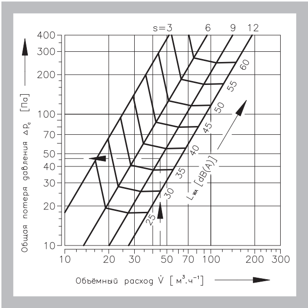
Диагр. 6.1.1. PVM-E90, размер 100
