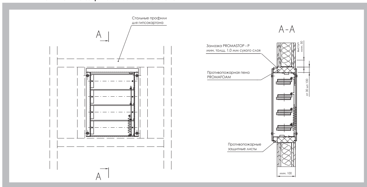
Рис. 13 Способ монтажа в жестких или гипсокартонных стеновых конструкциях - противопожарная пена PROMAFOAM-C закрыта замазкой PROMASTOP-P
