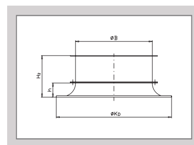
Самостоятельная передняя панель (без присоединительной коробки)
