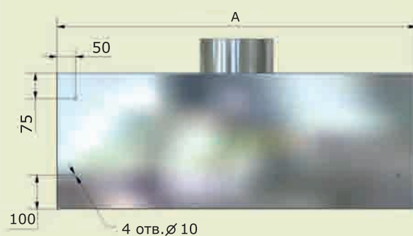
МВО - (А) МС (МСВ) - 08М х (В) Расположение отверстий для крепления к стене. Вид сзади.
