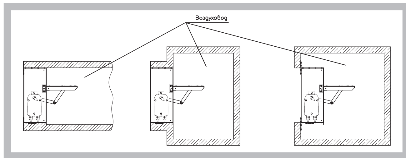
Рис. 10 Примеры установки клапанов «стенового» исполнения в горизонтальной плоскости
