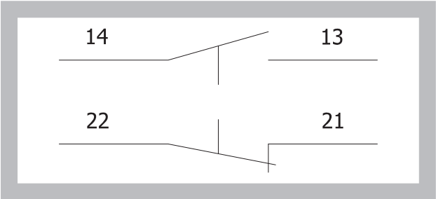
Рис. 12 Концевой выключатель ХСКН2118G-11
