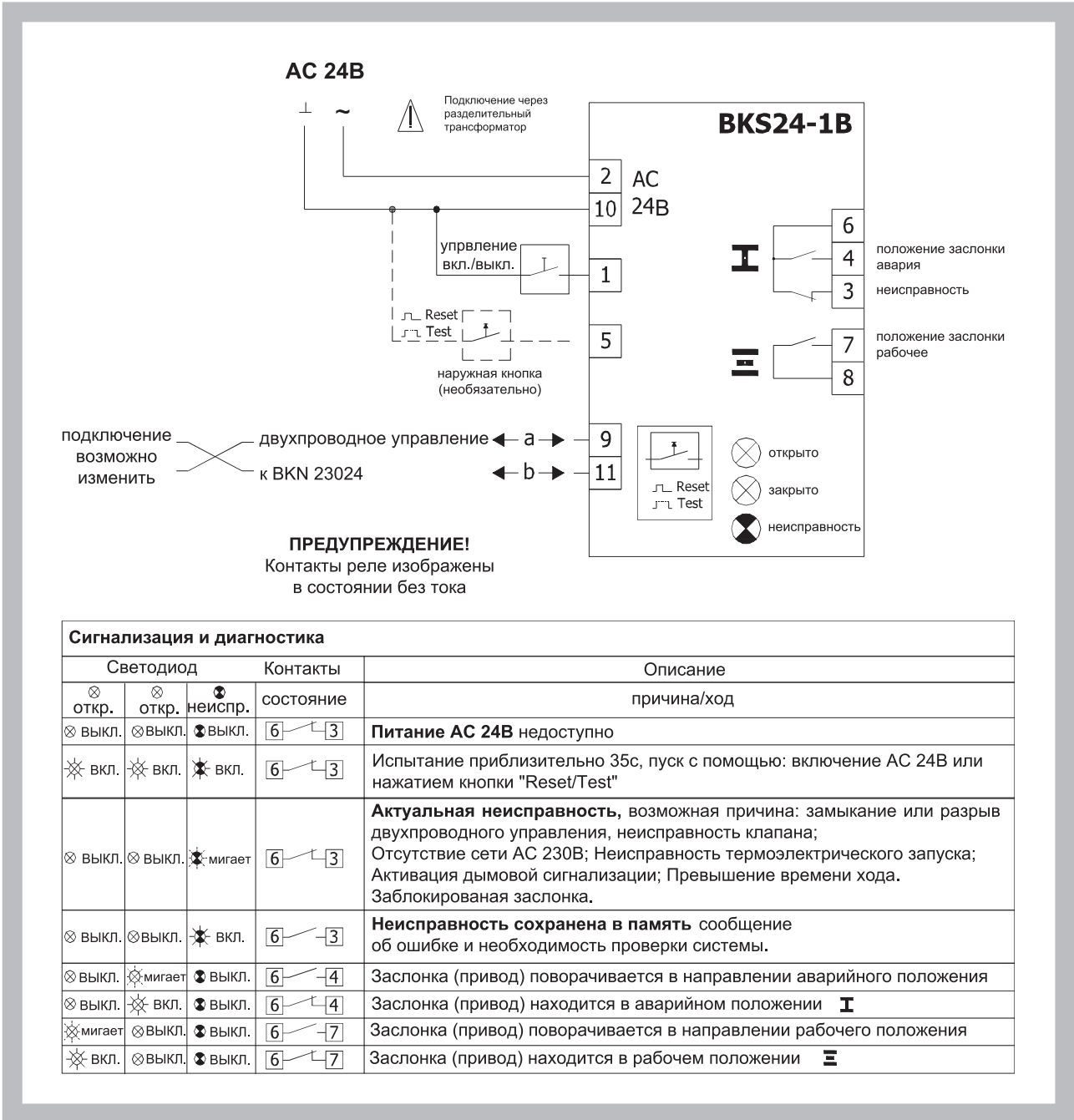
Рис. 39. Коммуникационное и управляющее устройство BKS 24-1B
