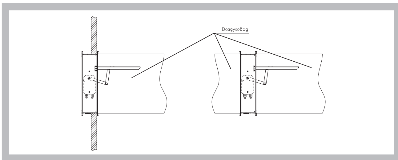
Рис. 11 Примеры установки клапанов «канального» исполнения
