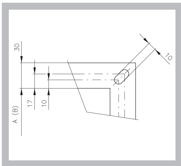
Рис. 6 Фланцы прямоугольного клапана
