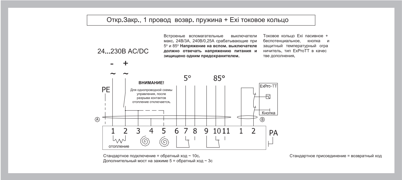
Рис. 35. Сервопривод Schischek ExMax-15-BF
