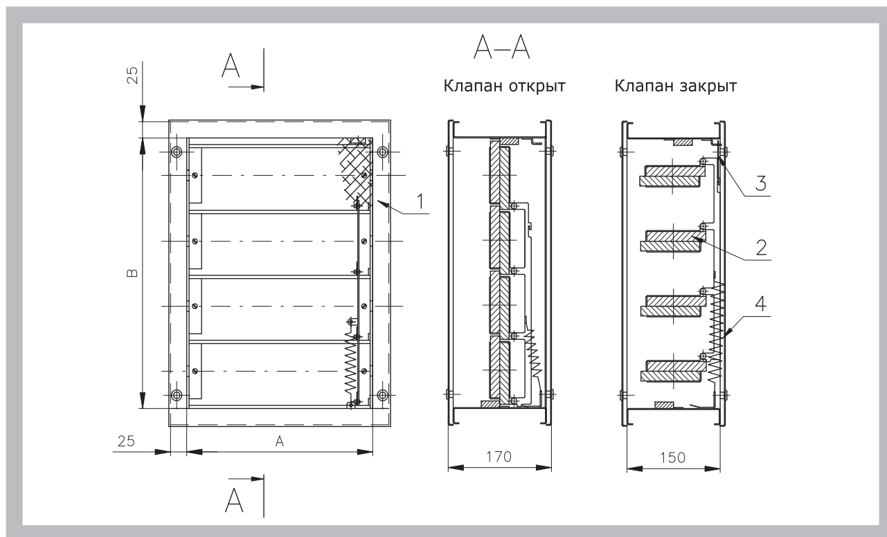
Рис. 3 Исполнение с сервоприводом
