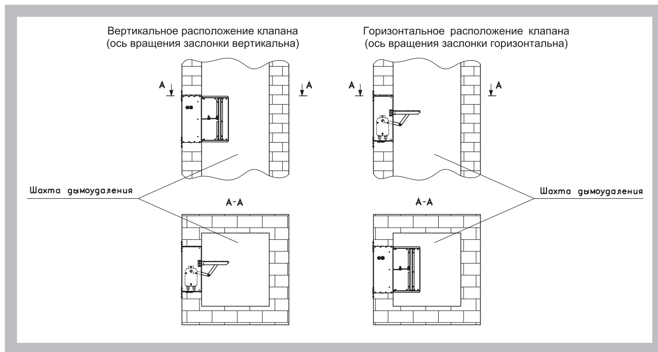
Рис. 9 В торце или на ответвлении воздуховода
