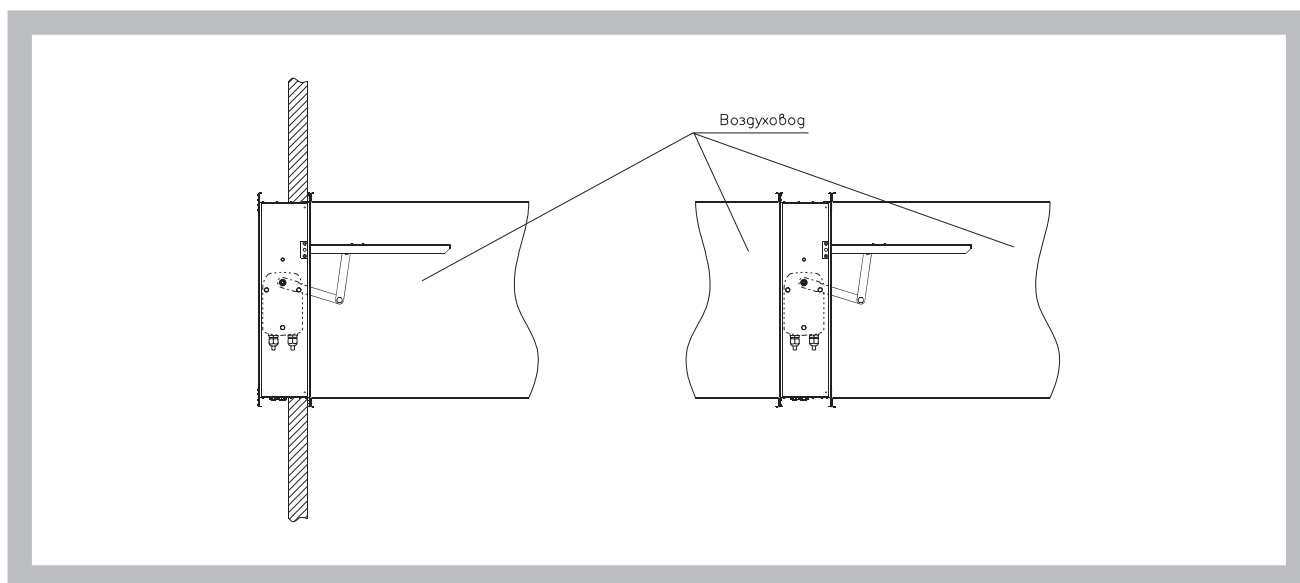
Рис. 11 Примеры установки клапанов «канального» исполнения
