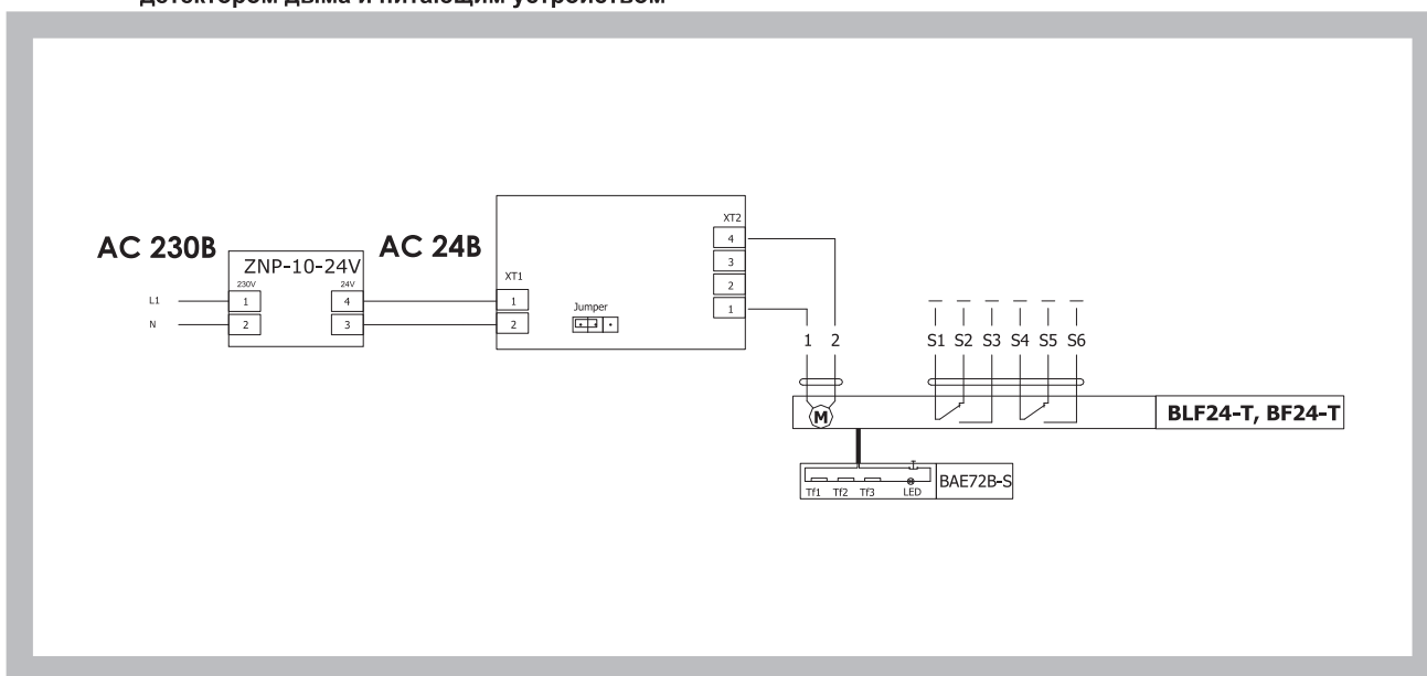
Рис. 26 Блок-схема подключения PSUM-90 в исполнении .41 - с сервоприводом BLF 24 - Т (BF 24 - Т), оптическим детектором дыма и питающим устройством
