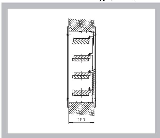
Рис. 18 Жесткая стеновая конструкция толщ. > 150 мм
