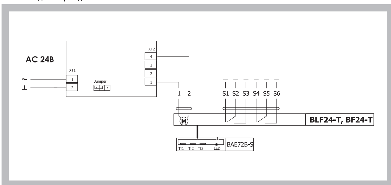
Рис. 27 Блок-схема подключения PSUM-90 в исполнении .51 - с сервоприводом BLF 24 - Т (BF 24 - Т) и оптическим детектором дыма
