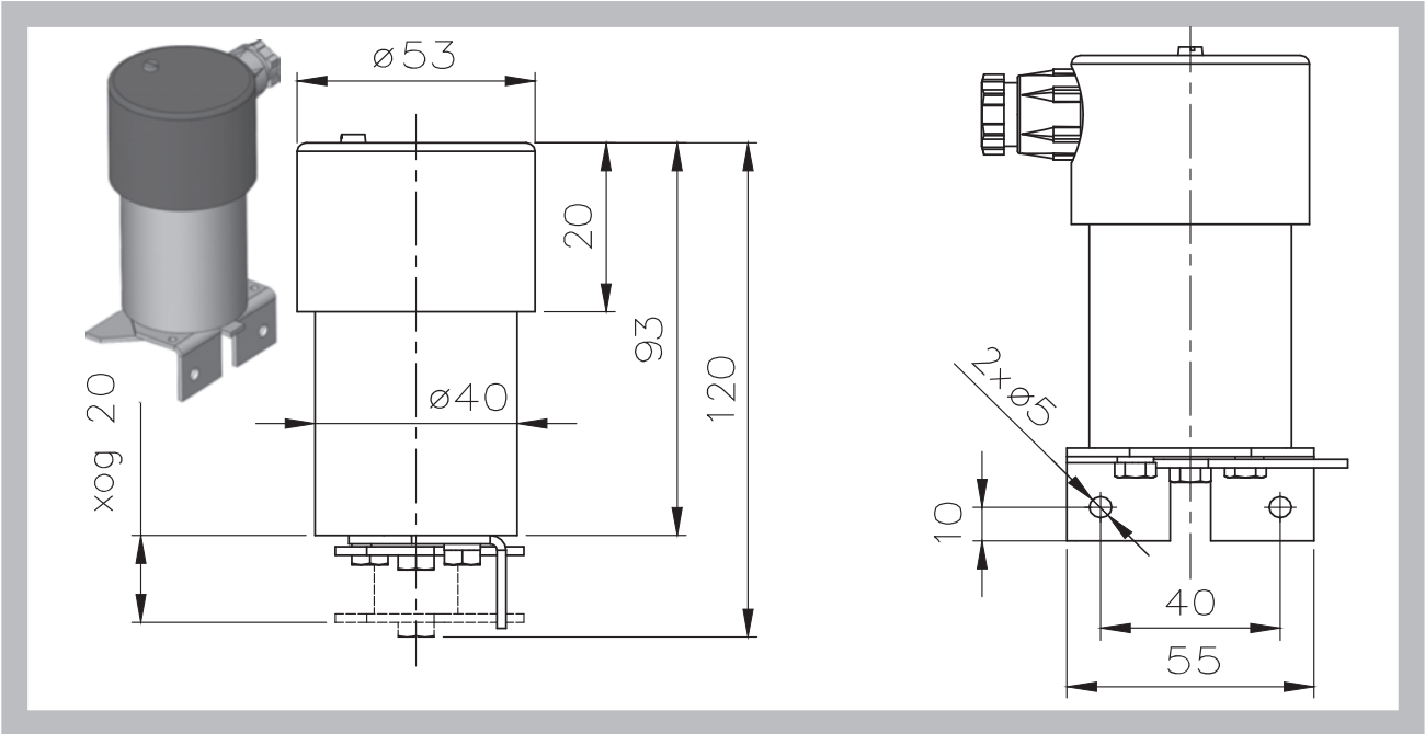
Рис. 14 Электромагнит EM230
