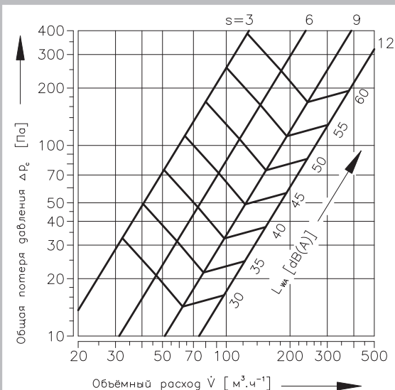
Диagr. 6.1.4. PVM-E90, размер 200
