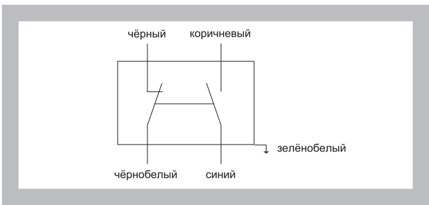
Рис. 26. Концевой выключатель XCW - A 115
