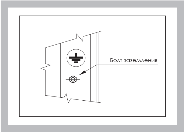
Рис. 19 Заземление клапана
