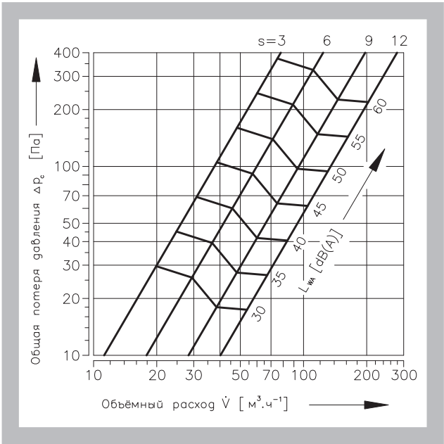
Диагр. 6.1.2. PVM-E90, размер 125
