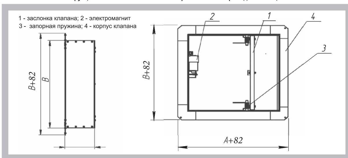
Рис. 3.2. Схема конструкции клапана ОКМ EI-90 с электромагнитным приводом и концевым выключателем
