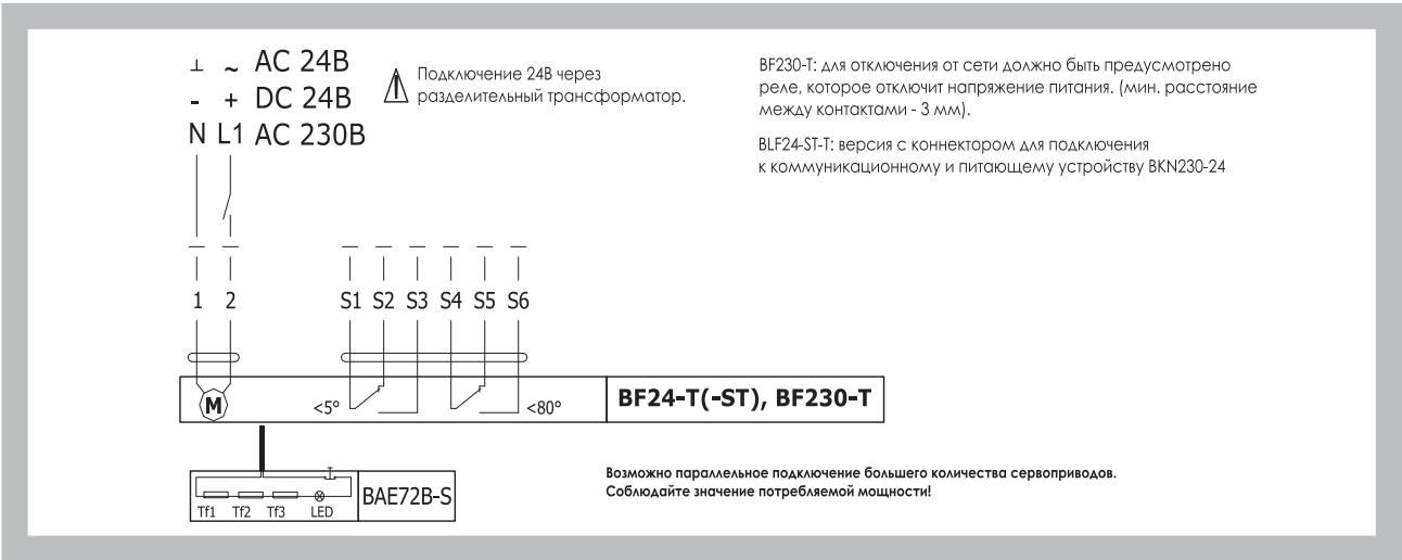
Рис. 24 Сервопривод BELIMO BF 24-T, BF 230-T
