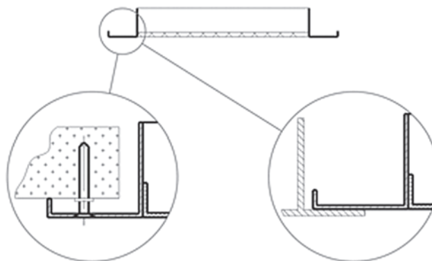
Монтаж с помощью открытого винтового крепления (для решеток РВС8)
