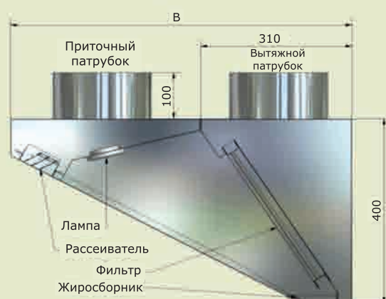
МВО - (А) МС -08 x (В) Устройство
