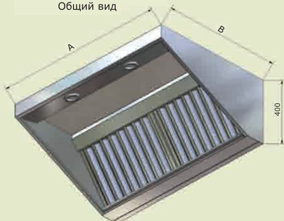
МВО - (А) МСВ - 08 х (В) Общий вид
