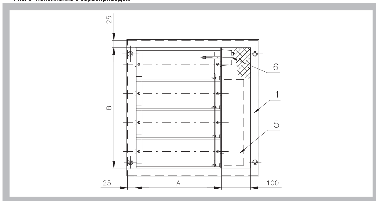
Рис. 3 Исполнение с сервоприводом
