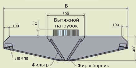
МВО - (А) МСВ -07С х (В) Устройство
