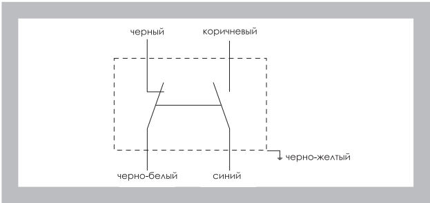
Рис. 21 Концевой выключатель XCW - A 115
