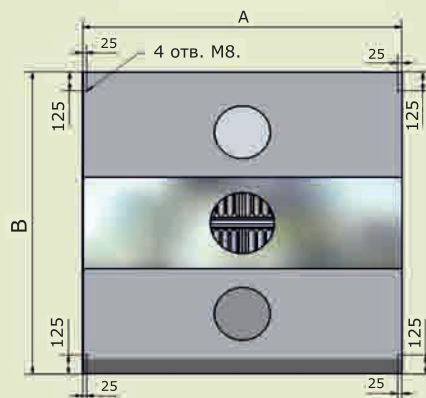
МВО - (А) МС - 07С х (В) Расположение отверстий для подвески к потолку. Вид сверху.
