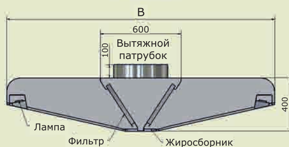
МВО - (А) МСВ -07СО х (В) Устройство
