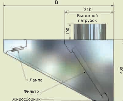
МВО - (А) МСВ - 08 х (В) Устройство
