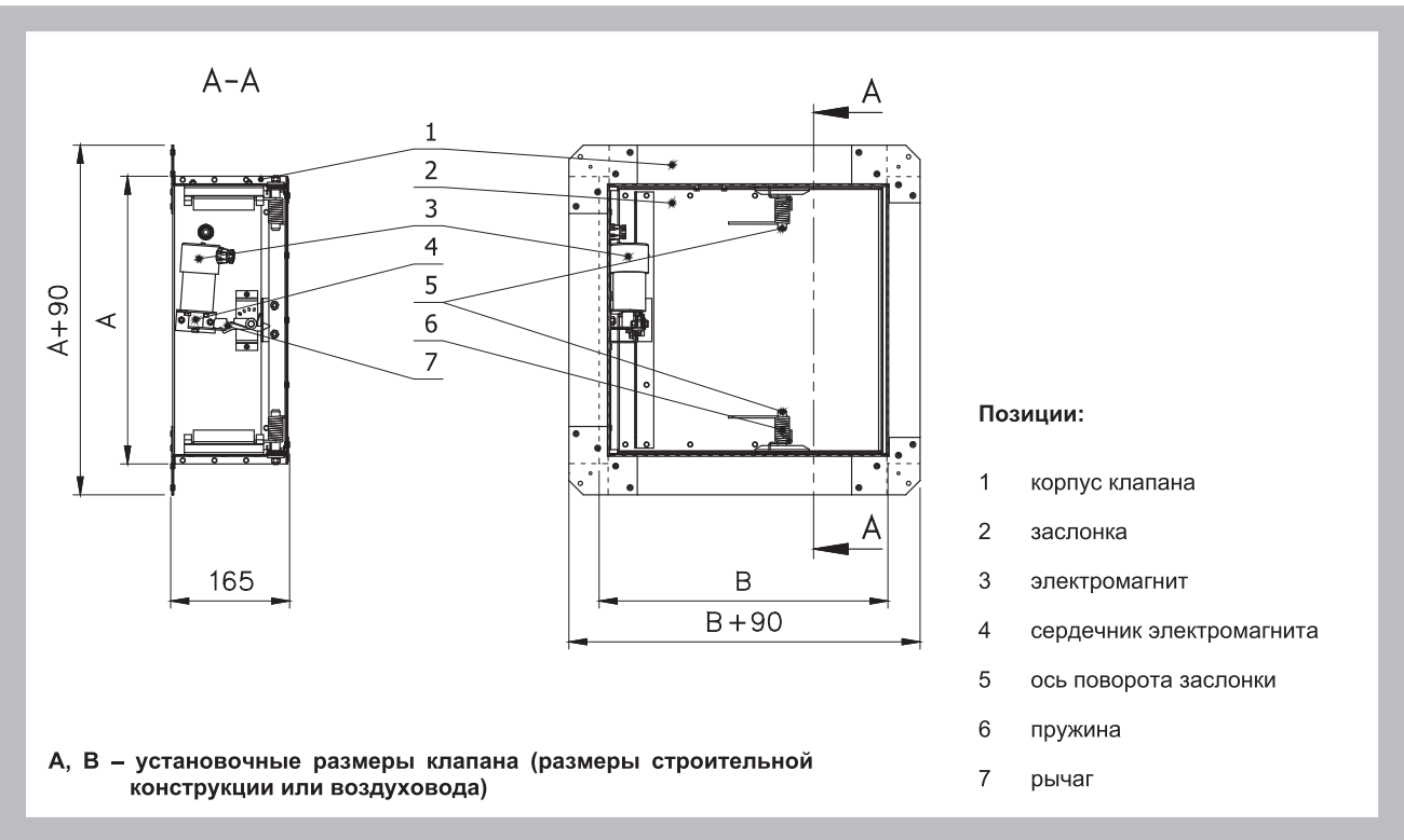
Рис. 2 Схема конструкции клапана ОКМ - Е-90 с электромагнитным приводом
