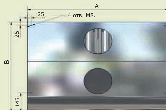
МВО - (А) МС (МСВ) - 08М х (В) Расположение отверстий для подвески к потолку. Вид сверху.
