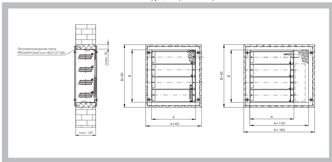
Рис. 12 Способ монтажа в жесткие стеновые конструкции - противопожарная пена PROMAFOAM-C или HILTI CP 620
