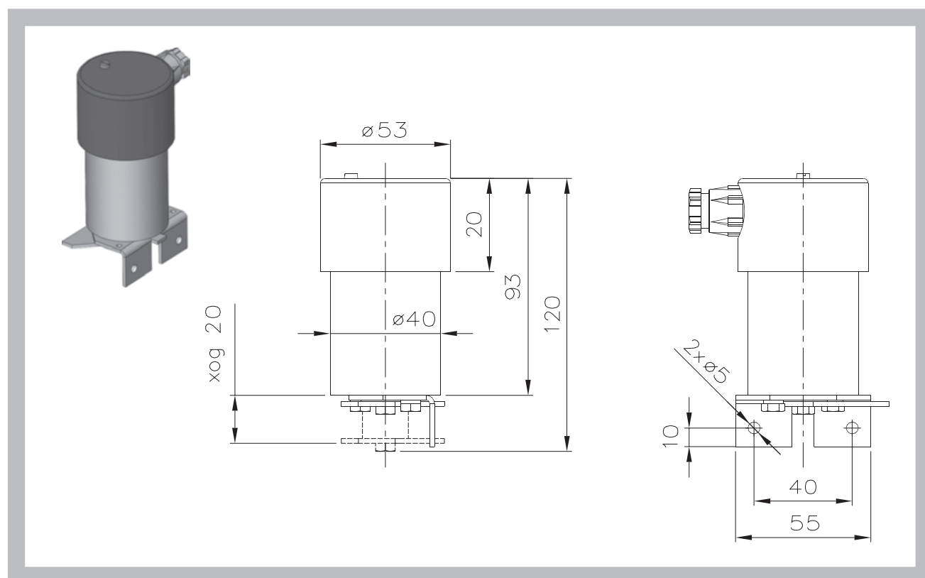
Рис. 14 Электромагнит EM230
