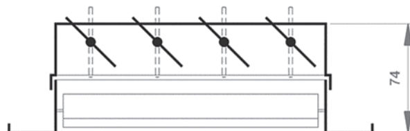
Регулируемая вентиляционная решетка РВС2-Б2, РВА2-Б2 (с клапаном Б2)
