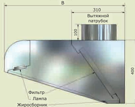
МВО - (А) МСВ - 08М х (В) Устройство
