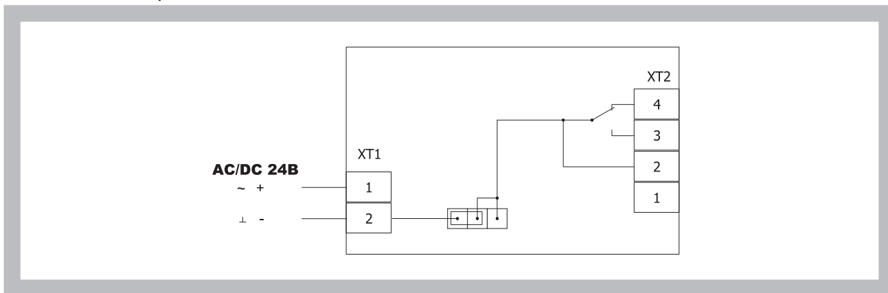
Рис. 25 Коннектор МНУ 734.031
