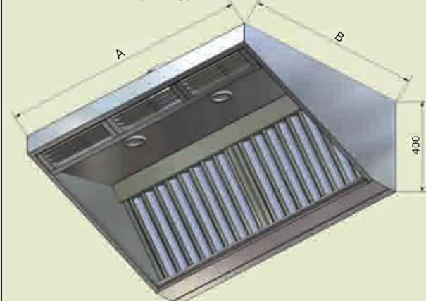
МВО - (А) МС -08 x (В) Общий вид
