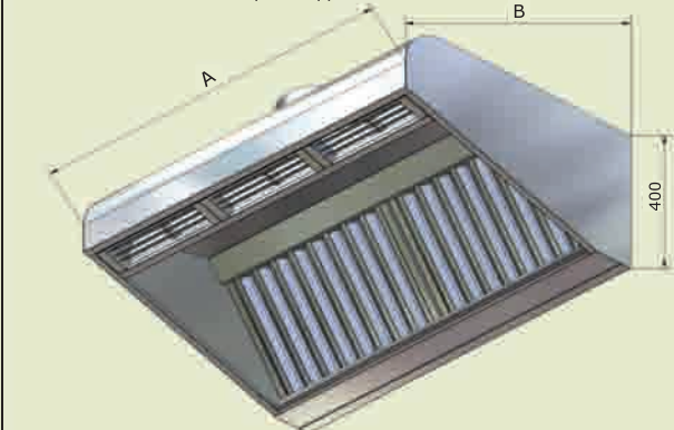
МВО - (А) МС -08М x (В) Общий вид
