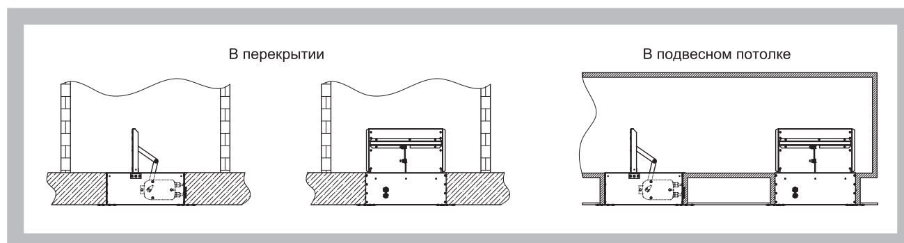
Рис. 10 Примеры установки клапанов «стенового» исполнения в горизонтальной плоскости
