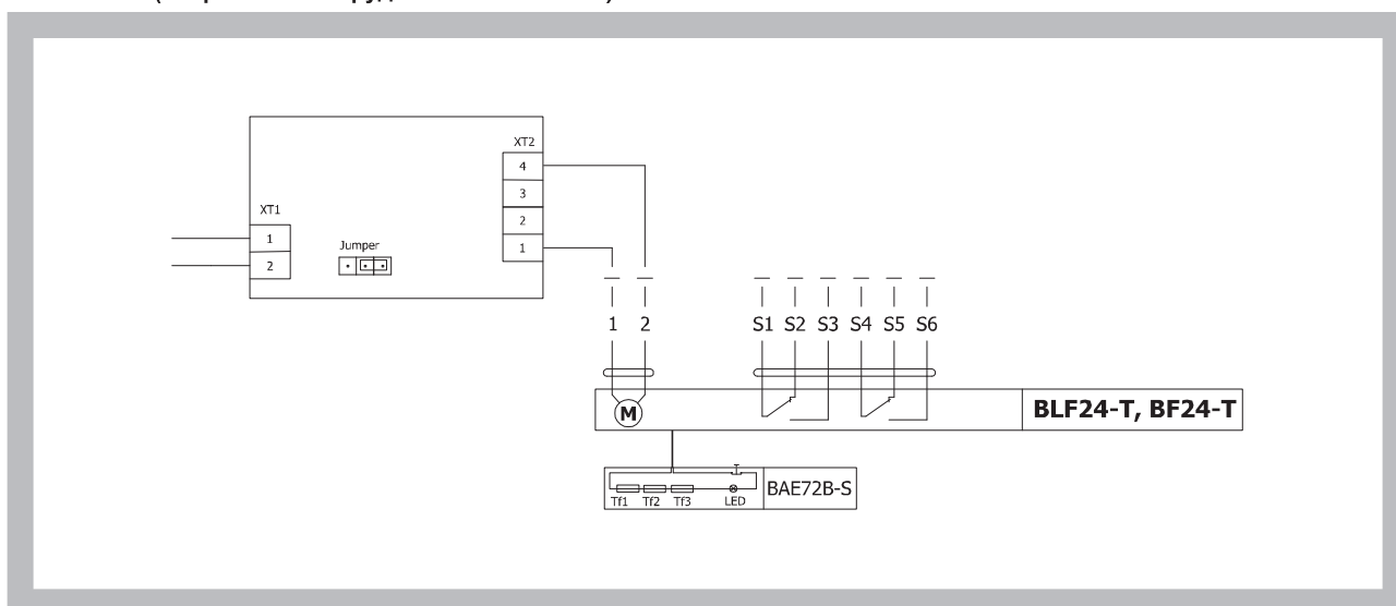
Рис. 43. Подключение с сервоприводом BF 24-T (BLF 24-T) и оптической дымовой сигнализацией HG 231 (напряжение оборудования AC/DC 24B)
