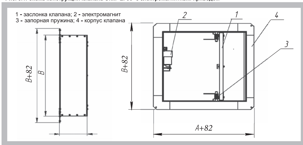
Рис. 3.1. Схема конструкции клапана ОКМ EI-90 с электромагнитным приводом
