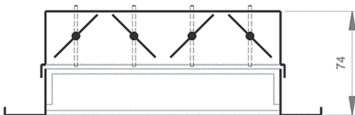
Конструкция нерегулируемой решетки РВА9 с клапаном Б1
