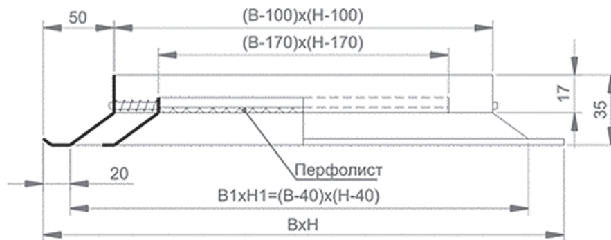
Конструкция потолочной вентиляционной решетки PBC5ПФ, PBA5ПФ
