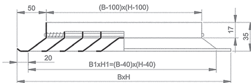
Конструкция потолочной вентиляционной решетки РВС5, РВА5
