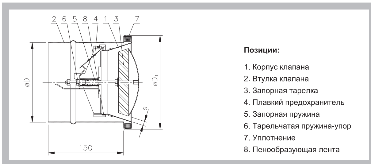
Рис. 2 Устройство клапана противопожарного PVM - E90 с электроприводом Belimo (установка электропривода перпендикулярно оси клапана) – Г – горизонтальная установка
