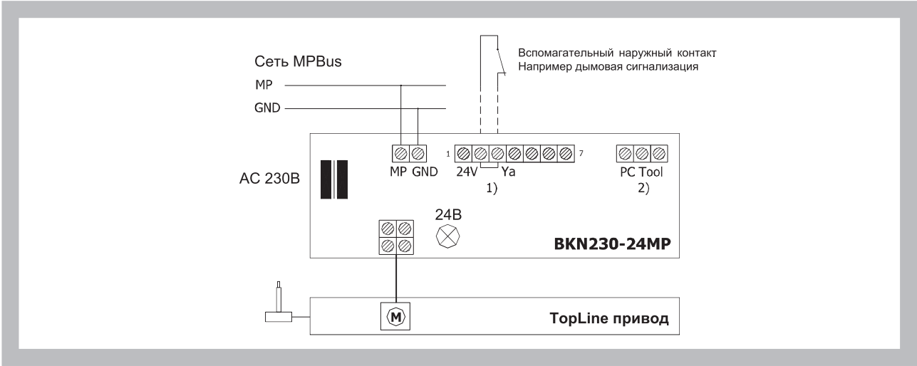
Рис. 37. Коммуникационное и управляющее устройство BKN 230-24MP
