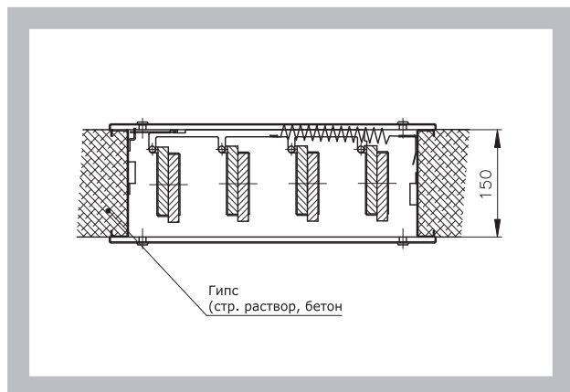
Рис. 6 Потолочная конструкция толщиной 150 мм
