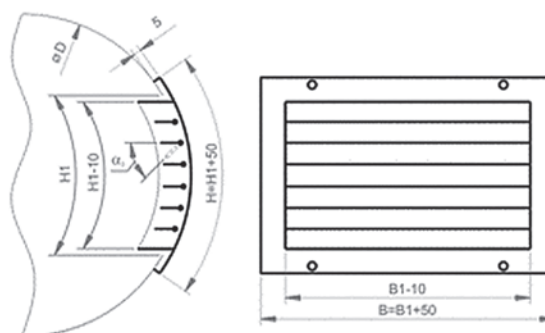
Конструкция решетки регулируемой РВС7
