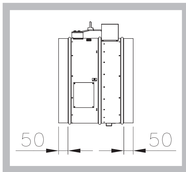
Рис. 7 Клапана для круглого воздухопровода
