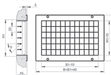
Регулируемая вентиляционная решетка РВС2-А, РВА2-А, РВН2-А
