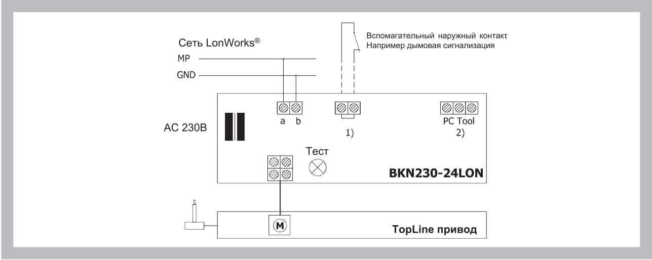
Рис. 38. Коммуникационное и управляющее устройство BKN 230-24LON
