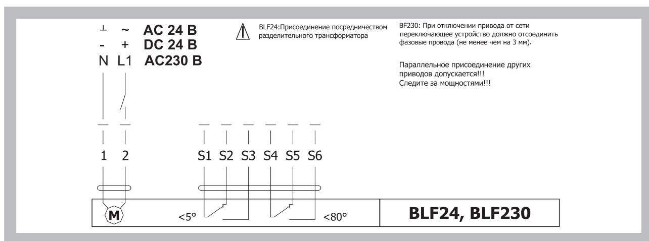
Рис. 4 Схема подключение электропривода BELIMO BLF 24, BLF 230
