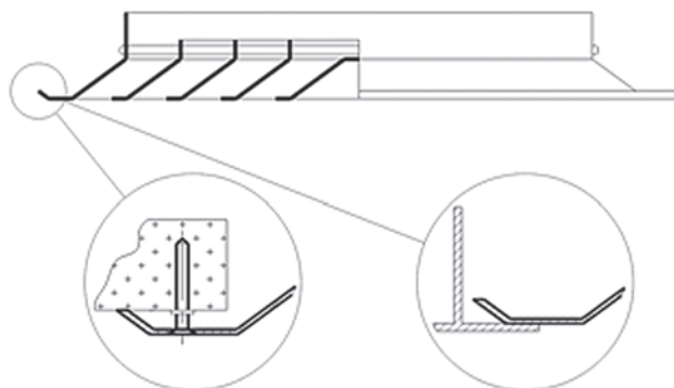
Монтаж с помощью открытого винтового крепления
