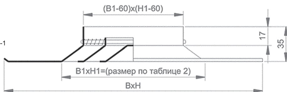
Конструкция потолочной вентиляционной решетки РВС5ПН, РВА5ПН
