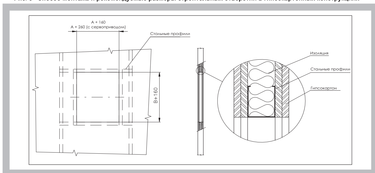
Рис. 5 Способ монтажа и рекомендуемые размеры строительных отверстий в гипсокартонных конструкциях
