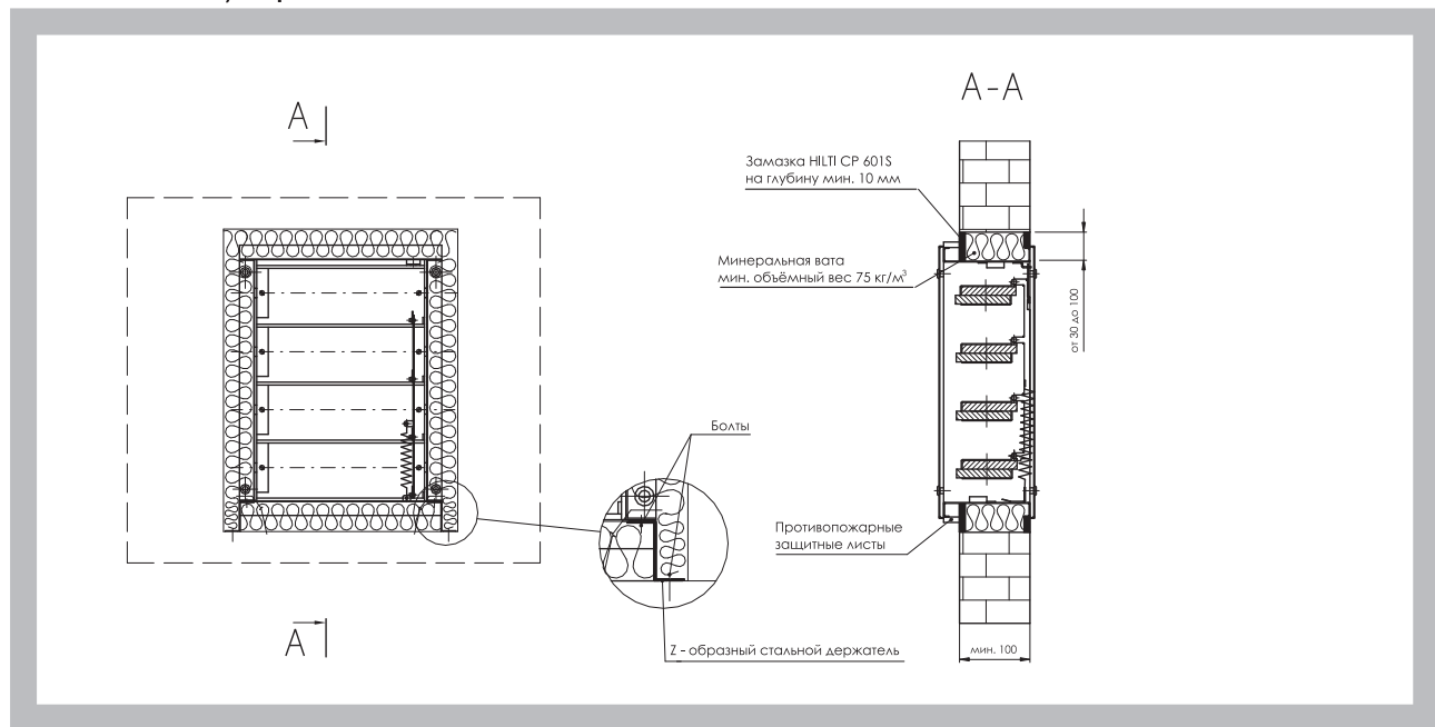
Рис. 15 Способ установки клапана в жестких стеновых конструкциях - минеральная вата (объемный вес мин. 75 \text{ кг/м}^3 ) закрыта замазкой HILTI CP 601S
