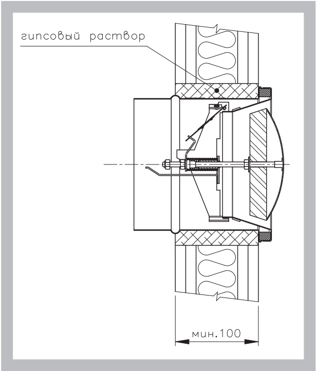
Рис. 5 Без присоединения к воздуховоду
