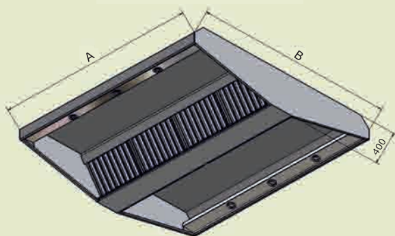
МВО - (А) МСВ -07С х (В) Общий вид
