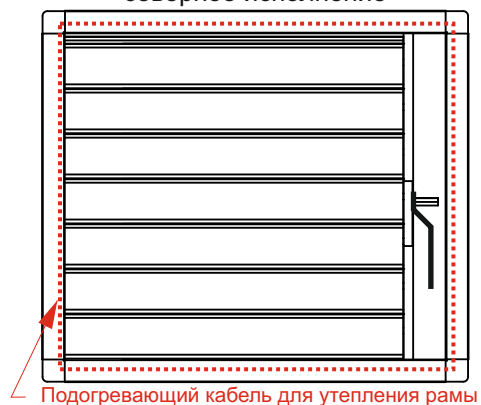
РЭД-УВК-Ст-ПП-Сев Стеновой с площадкой под привод северное исполнение
