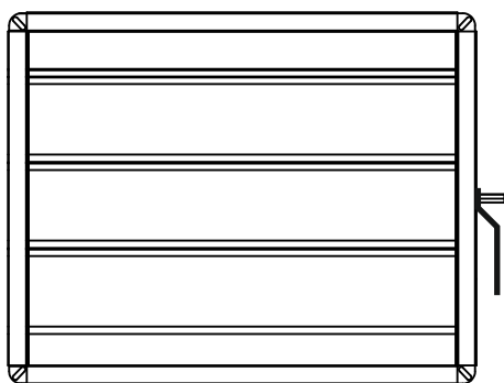
РЭД-УВК-Кан-Р Канальный с ручной регулировкой
