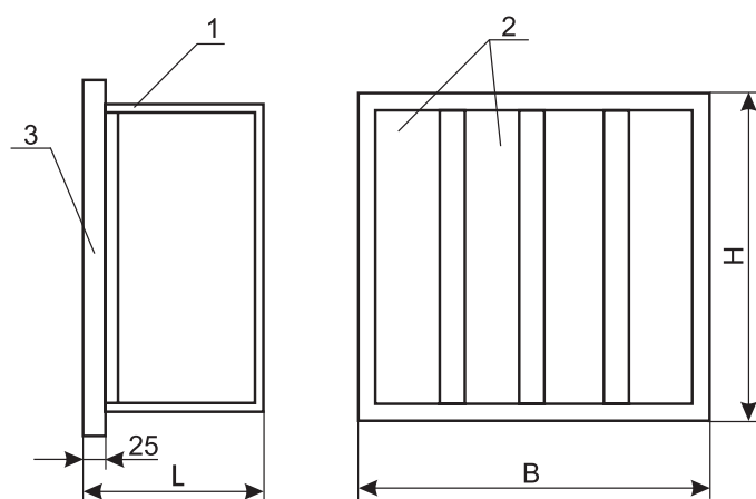
Рис. 1 Схема фильтра FYK-SP-K
