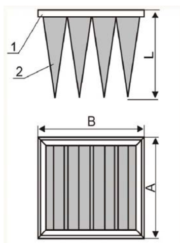
Рис. 1 Схема фильтра FYK-SP
