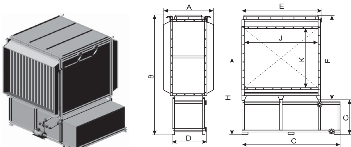
Рис.1 Монтажные и габаритные размеры фильтров RIF
