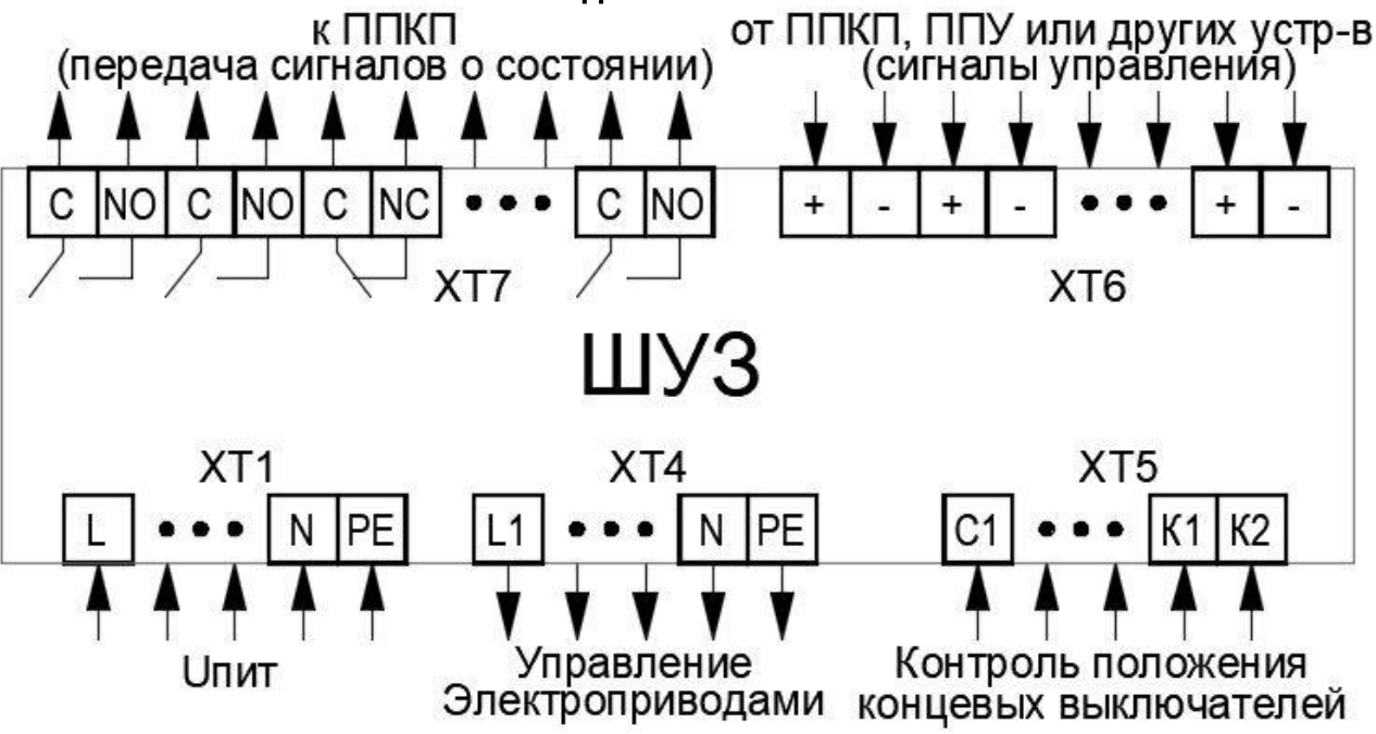
Схема внешних подключений для ШУЗ-1(1,1кВт; 230; 54; СП)
