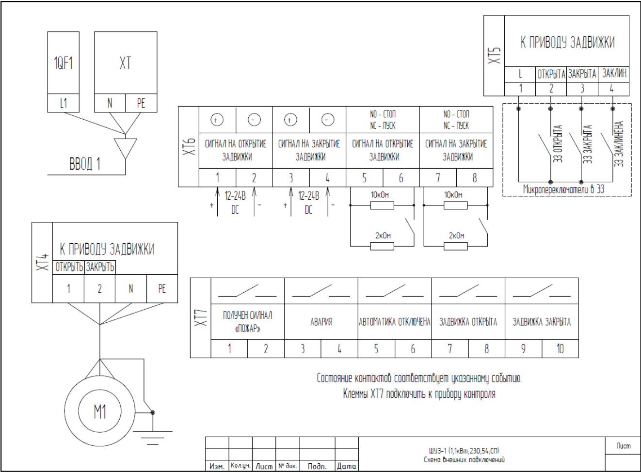
Схема внешних подключений для ШУЗ-1(1,1кВт; 230; 54; СП)
