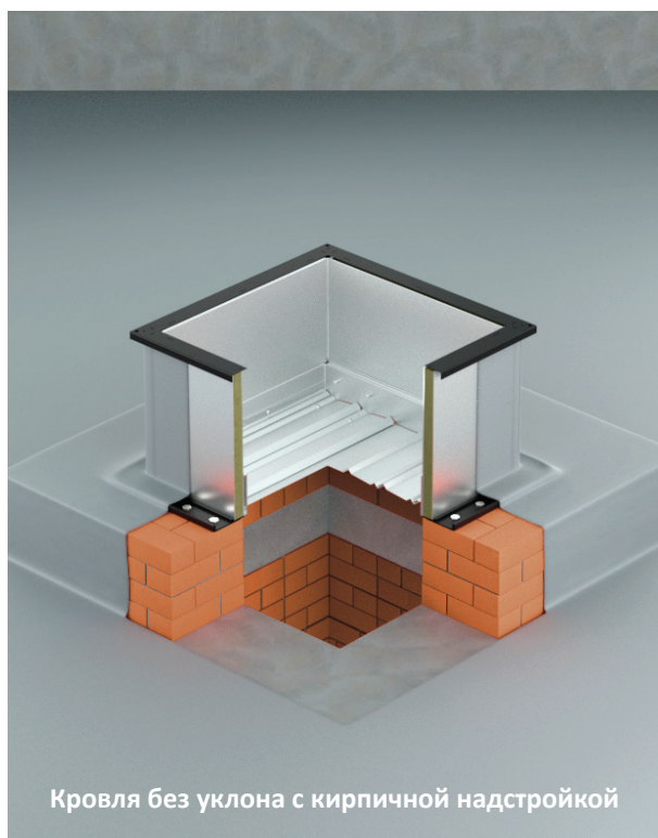
Модель стакана со встроенным обратным клапаном VO (вытяжка)
