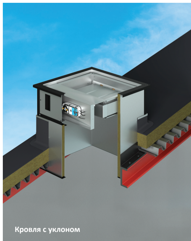
Модель обслуживаемого стакана со встроенным приводным обогреваемым клапаном DW
