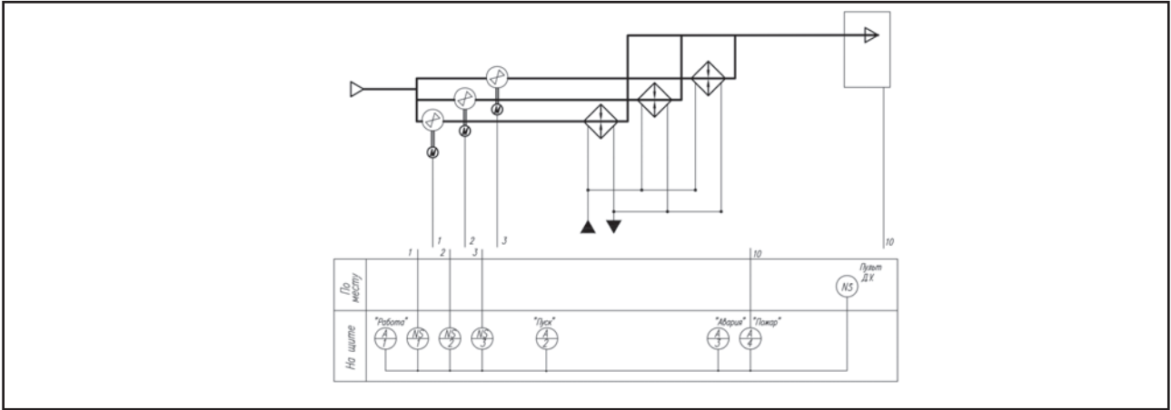
Схема электическая соединений АВО-К-1.3-3фазный
