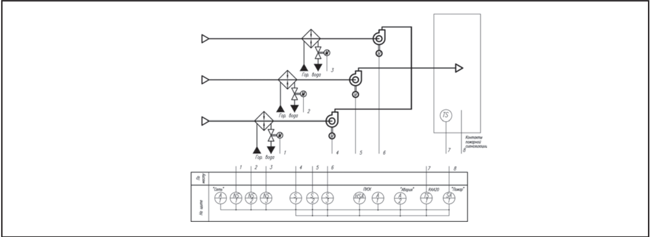
Схема электическая соединений АВО-К-2.3-3фазный
