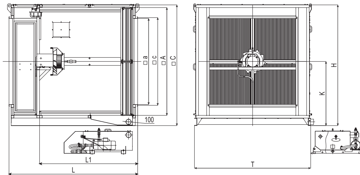
Рисунок 2. УФИН №№ 6,3...12,5
