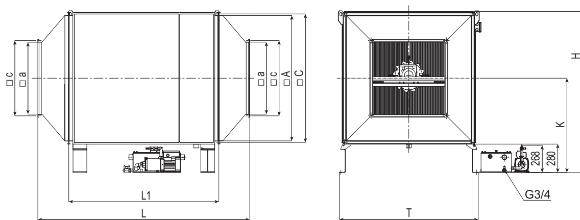
Рисунок 1. УФИН №№ 2...5
